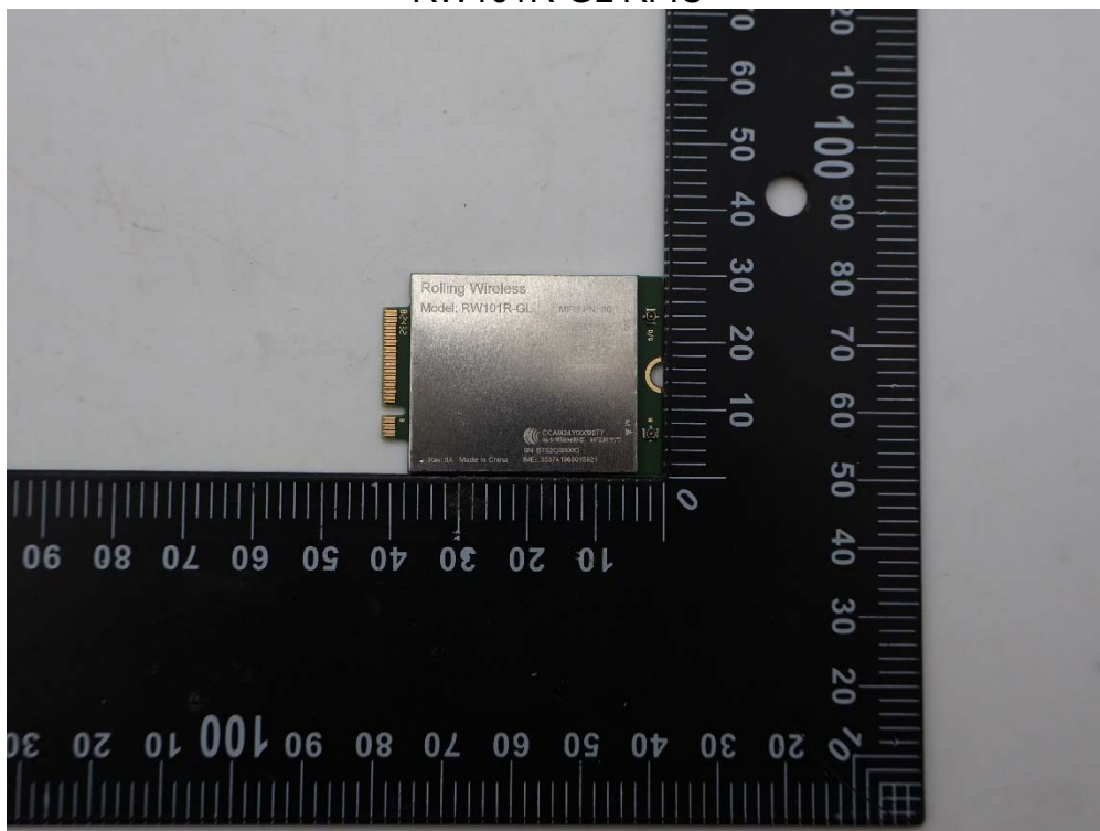
RW101R-GL RFIC
