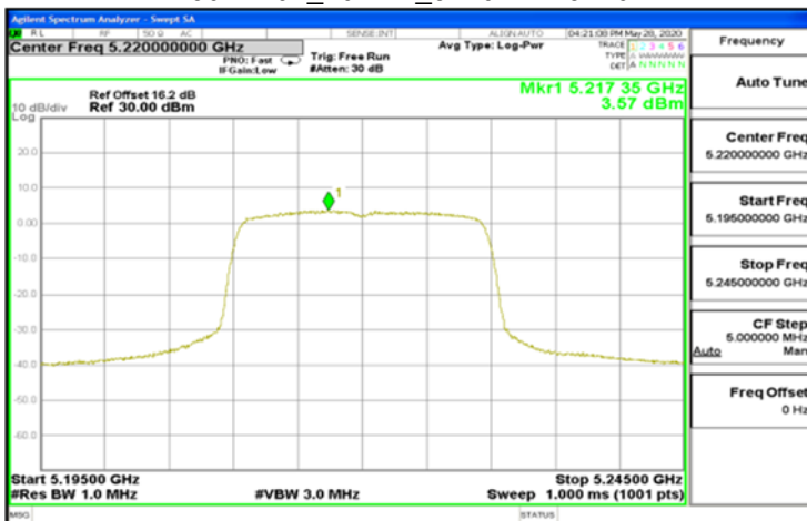
802.11ax_20MHz_5220MHz-5220
