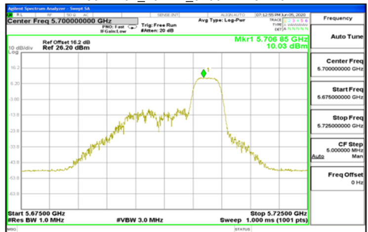
802.11ax_20MHz_5700MHz-52-40
