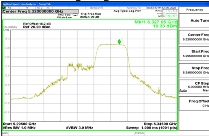
802.11ax_20MHz_5320MHz-26-8
