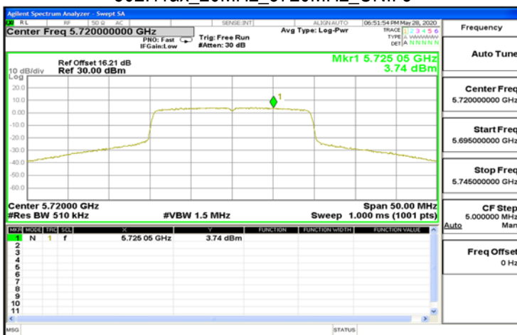
802.11ax_20MHz_5720MHz_UNII 3
