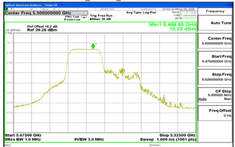
802.11ax_20MHz_5500MHz-26-0
