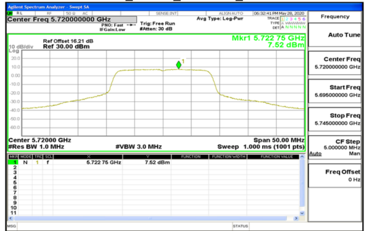
802.11a_20MHz_5720MHz_UNII 3
