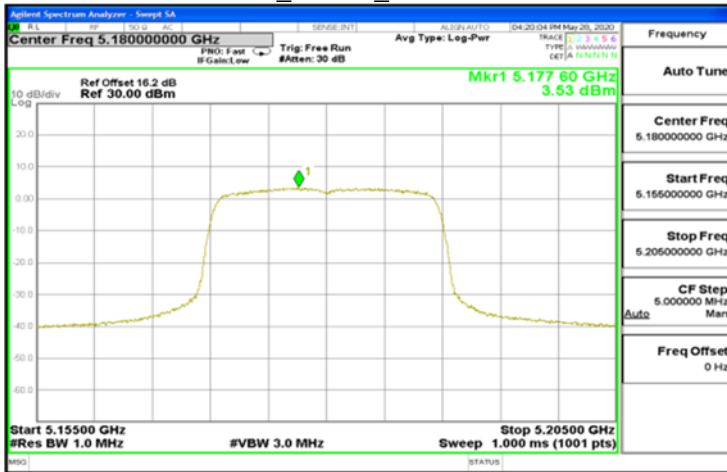
802.11ax_20MHz_5180MHz-52-37
