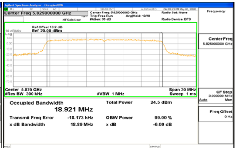
IC_802.11ax_20MHz_Chain1_5825MHz
