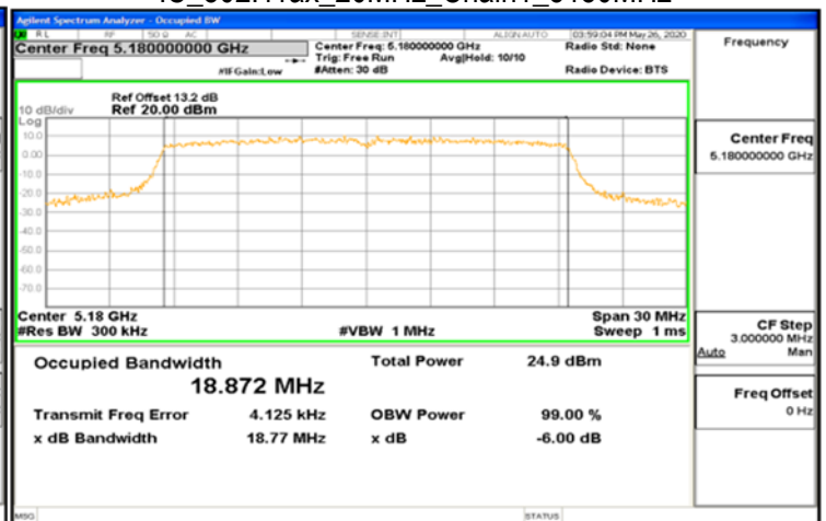
IC_802.11ax_20MHz_Chain1_5180MHz
