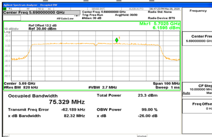
FCC_802.11ac_80MHz_Chain1_5690MHz
