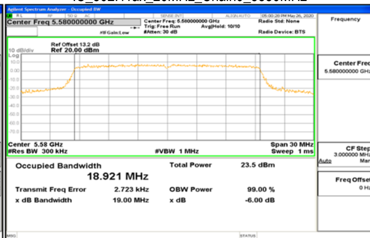
IC_802.11ax_20MHz_Chain0_5580MHz
