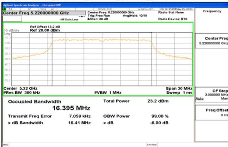
IC_802.11a_20MHz_Chain1_5220MHz
