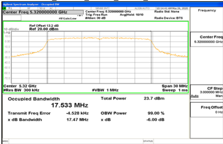
IC_802.11n_20MHz_Chain1_5320MHz
