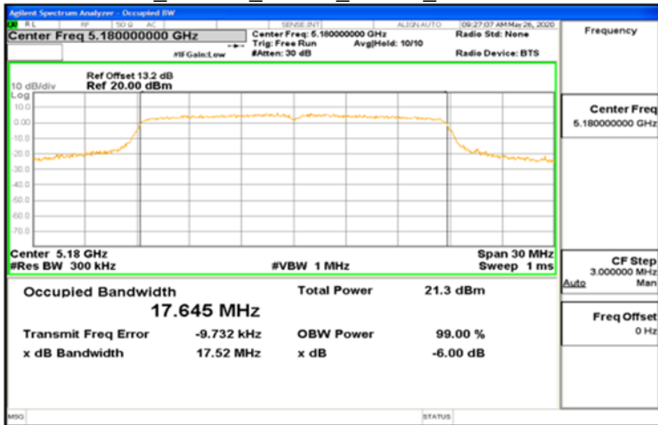
IC_802.11n_20MHz_Chain0_5180MHz
