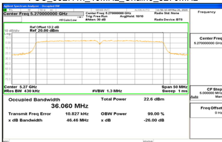
FCC_802.11n_40MHz_Chain0_5270MHz
