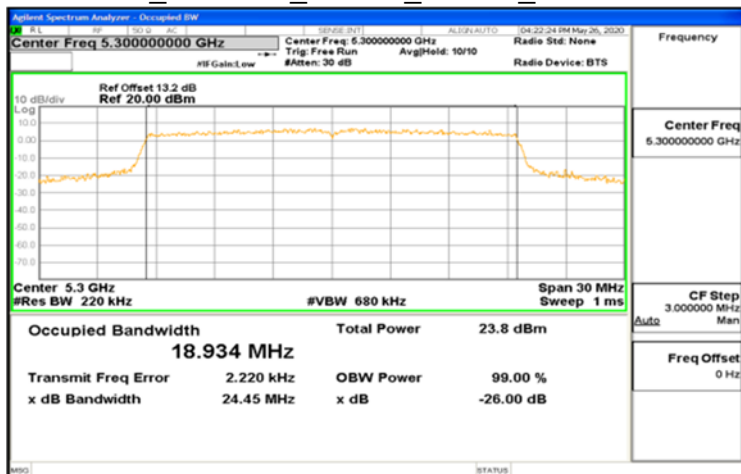
FCC_802.11ax_20MHz_Chain0_5300MHz
