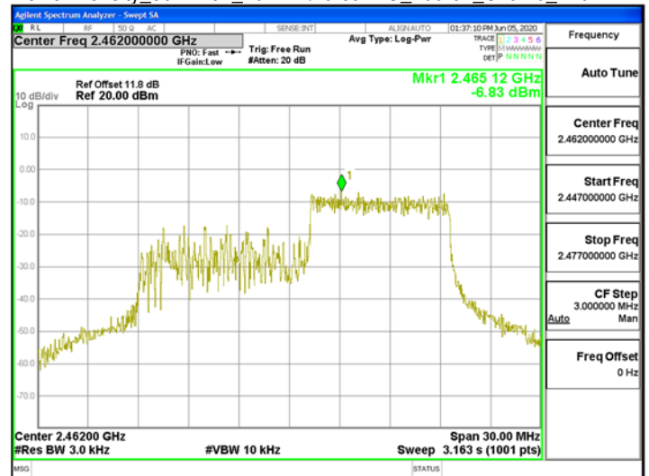
Power Density 802.11ax 20MHz\Partial RU 106-54 Chain1 2462MHz
