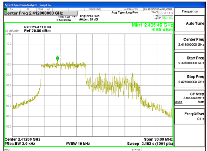
Power Density 802.11ax 20MHz\Partial RU 106-53 Chain1 2412MHz
