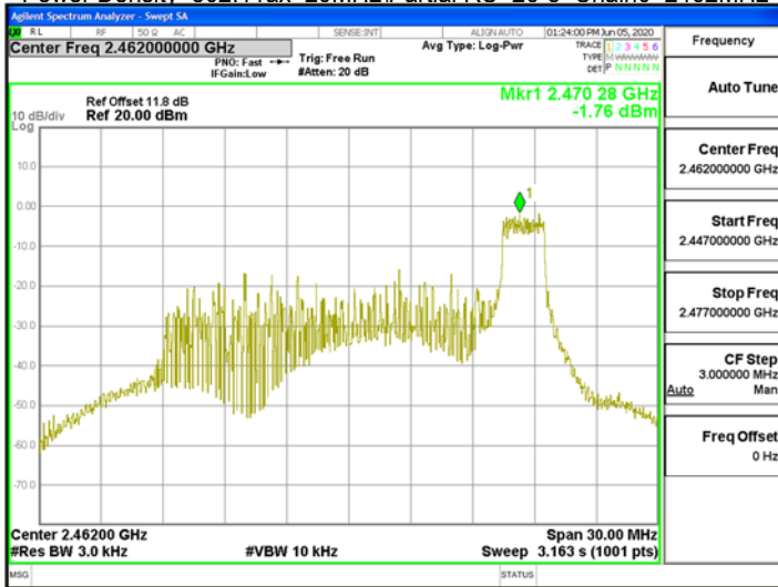
Power Density 802.11ax 20MHz\Partial RU 26-8 Chain1 2462MHz
