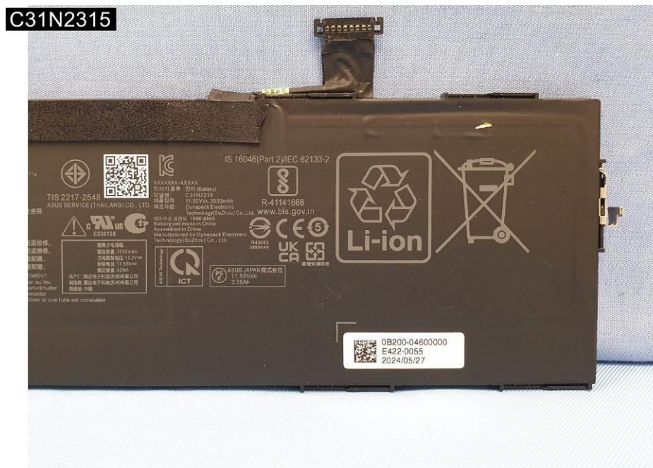
EUT Photo (12)
