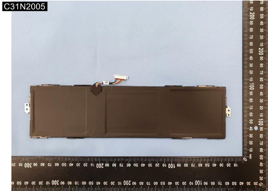
EUT Photo (18)
