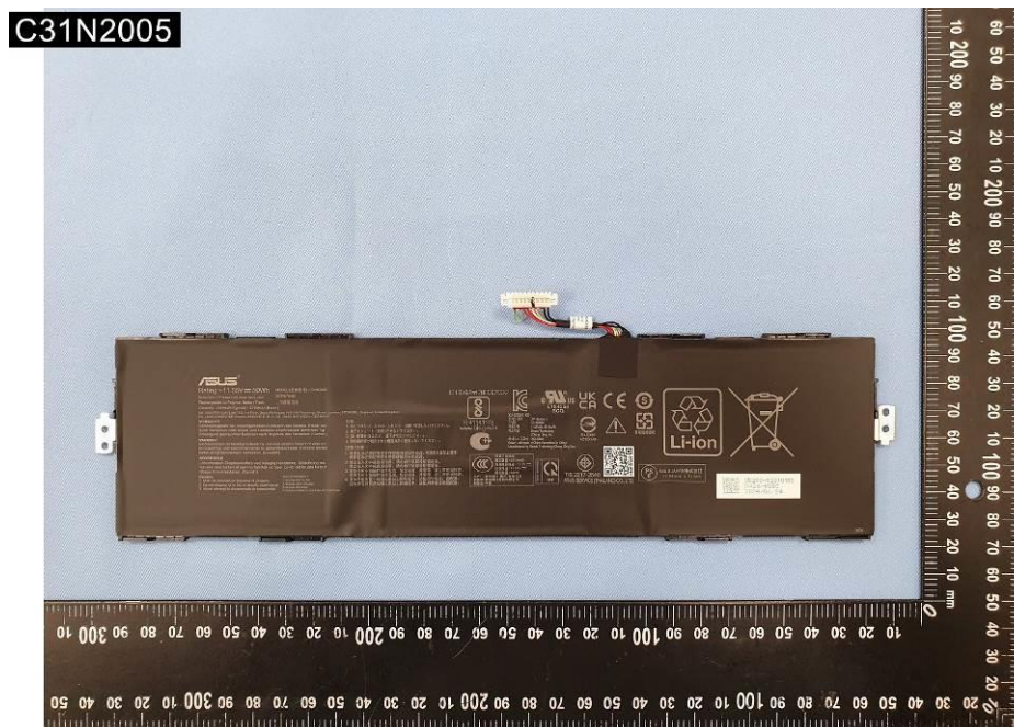
EUT Photo (14)
