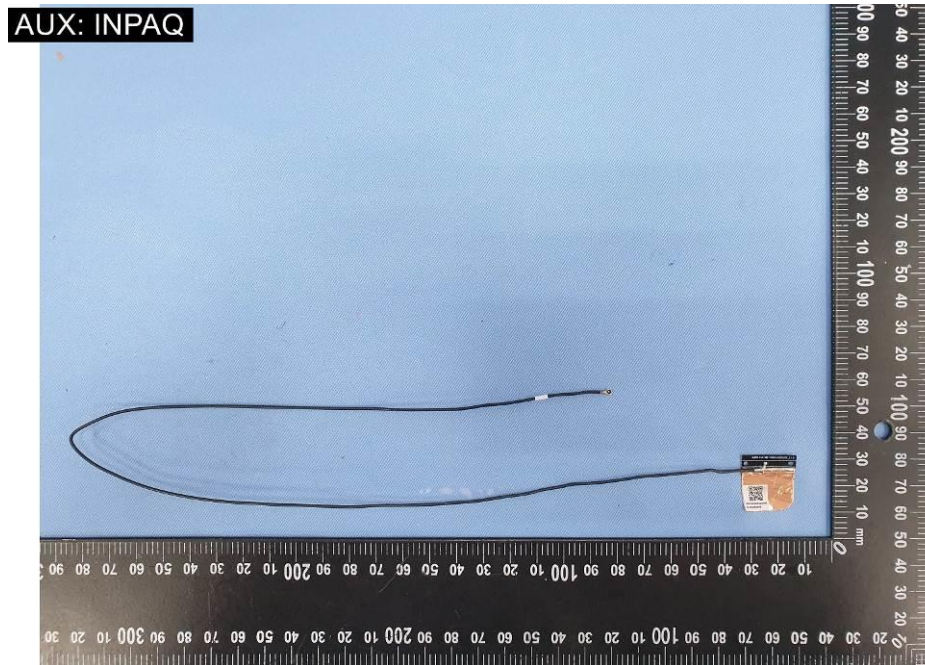
EUT Photo (18)
