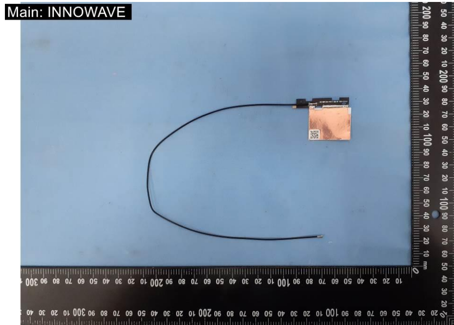
EUT Photo (20)
