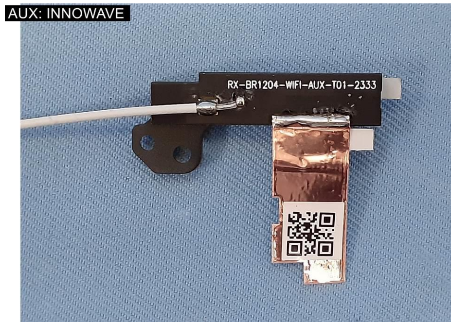
EUT Photo (24)
