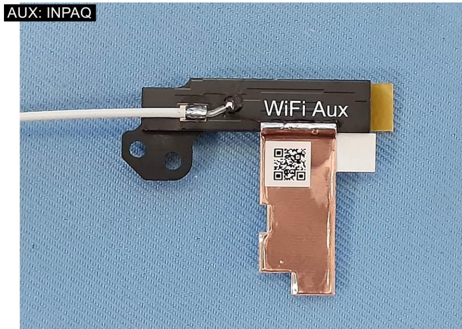
EUT Photo (16)
