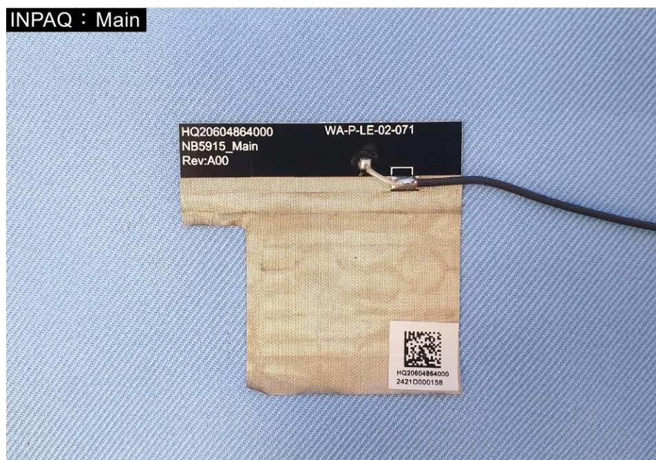
EUT Photo (40)
