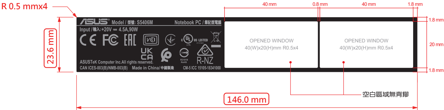
出標樣式/佈膠示意圖
