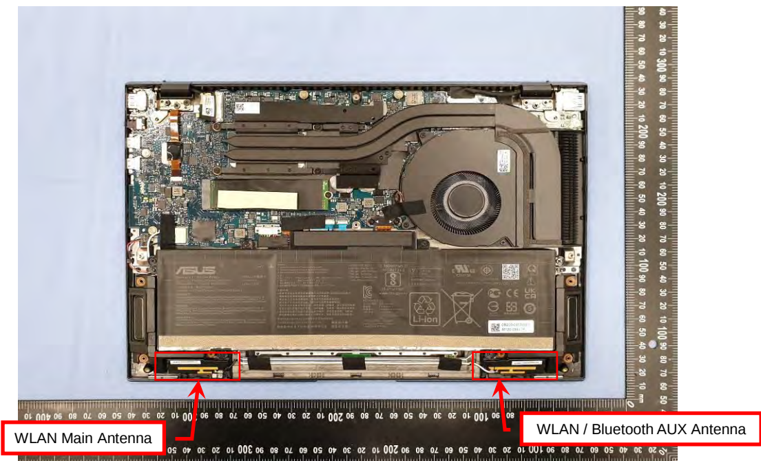
EUT Photo (2)
