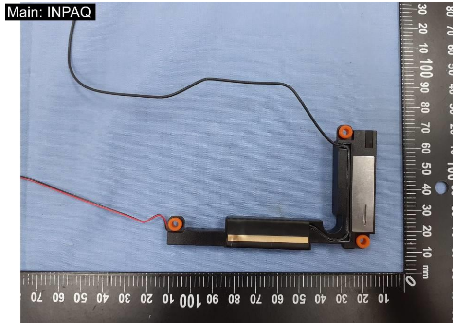
EUT Photo (31)
