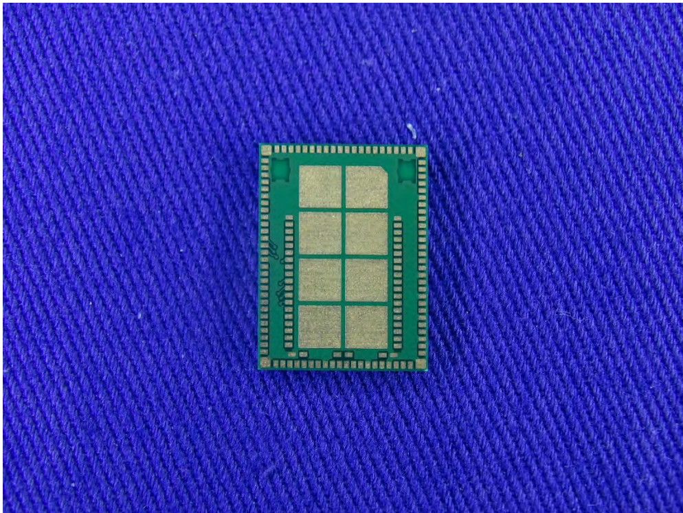
(67) EUT Photo
