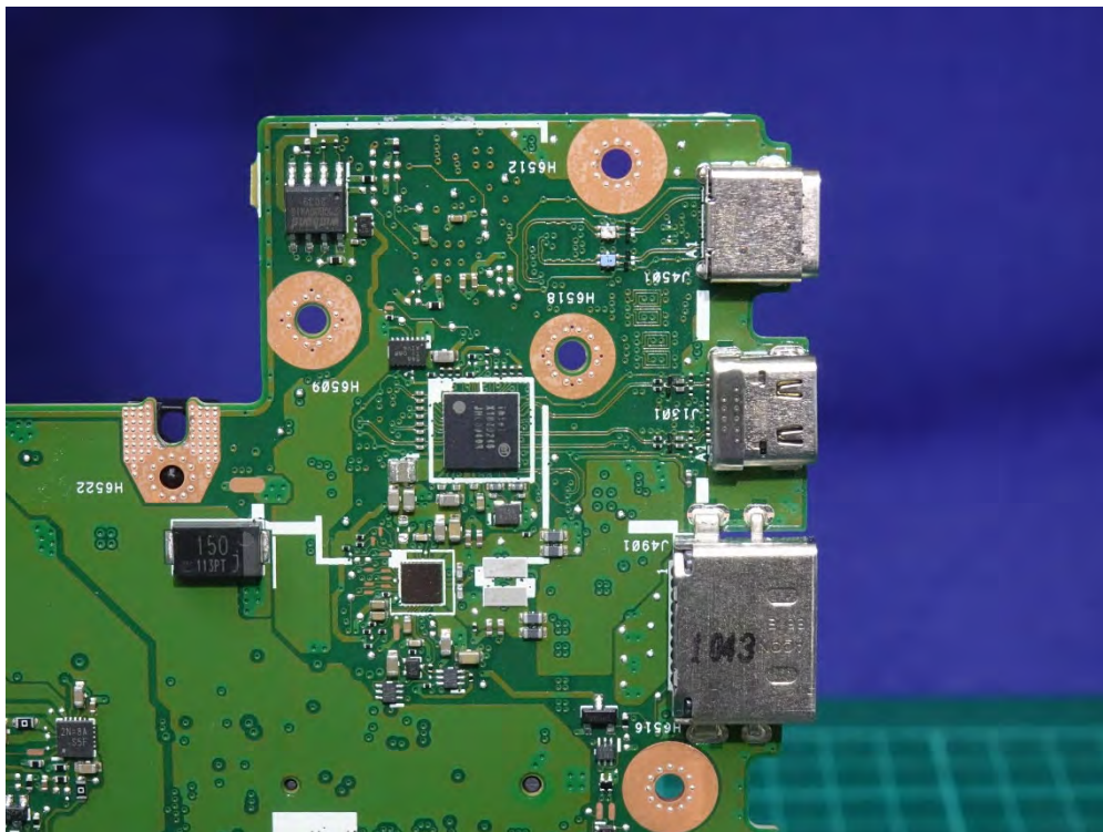
(59) EUT Photo
