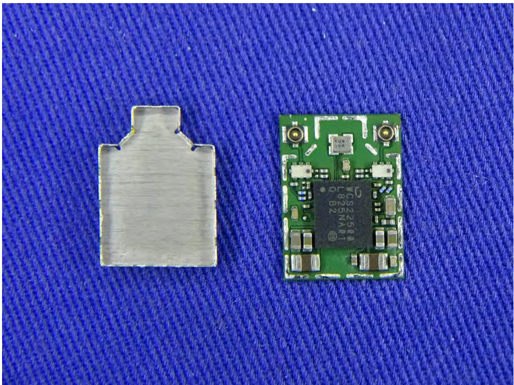
(65) EUT Photo
