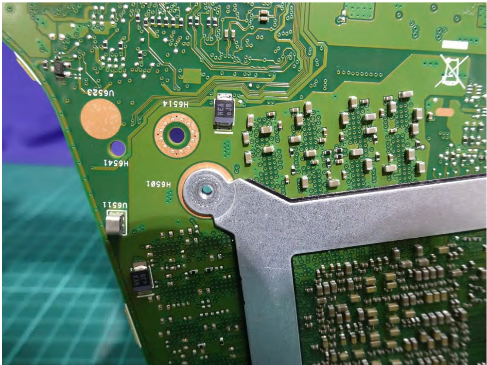
(54) EUT Photo
