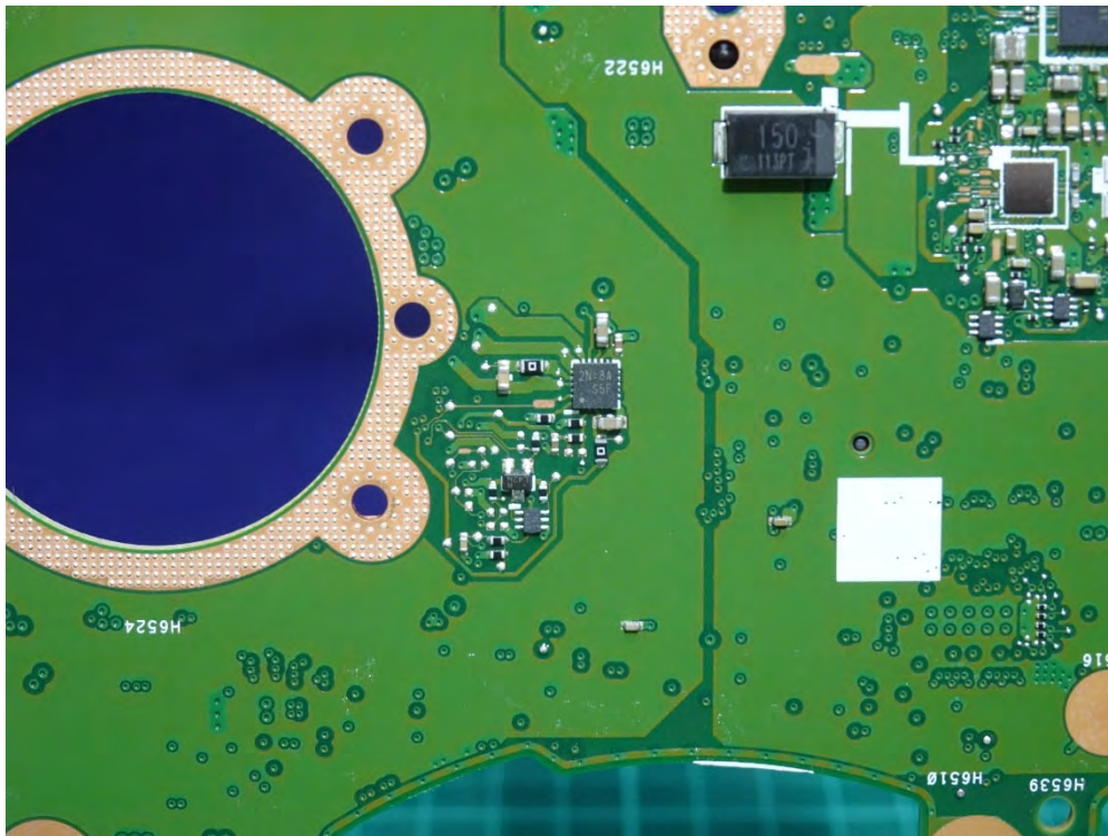
(58) EUT Photo
