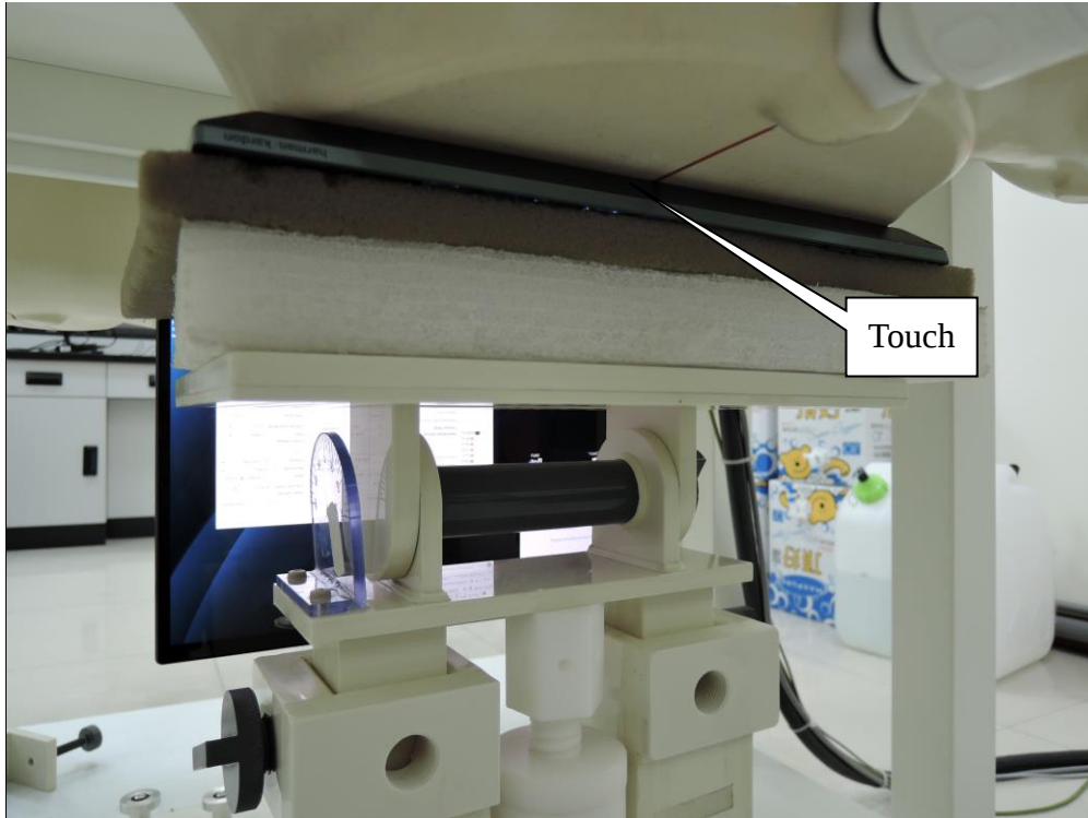
EUT Bottom (NB)
