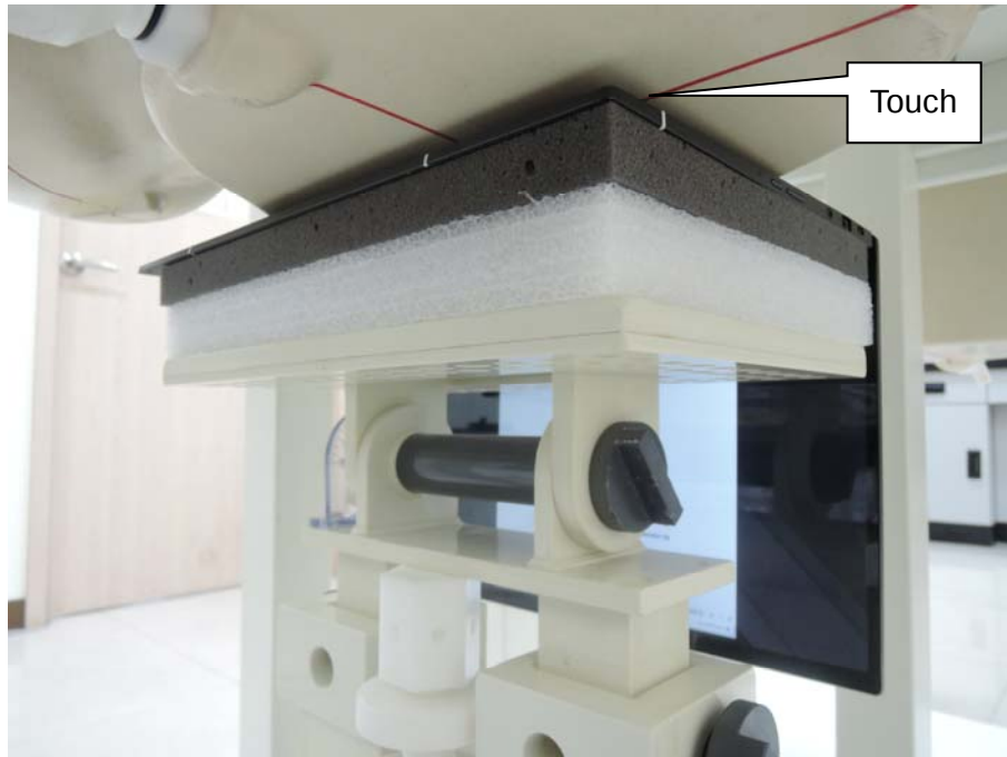
EUT Bottom (NB) - Main Antenna
