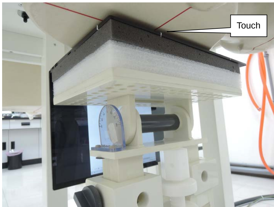
EUT Bottom (NB) - Aux Antenna
