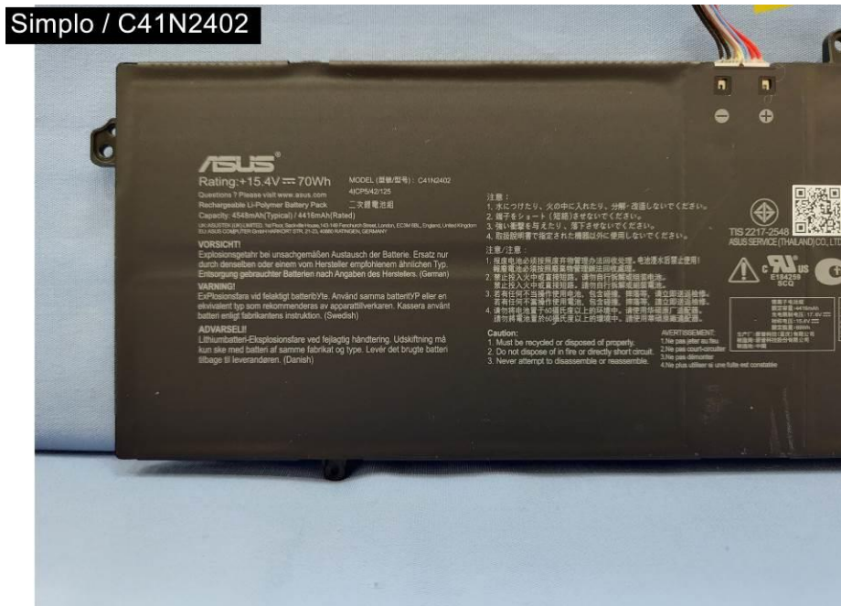
EUT Photo (10)
