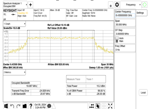
802.11be_20MHz_Chain0_6435MHz
