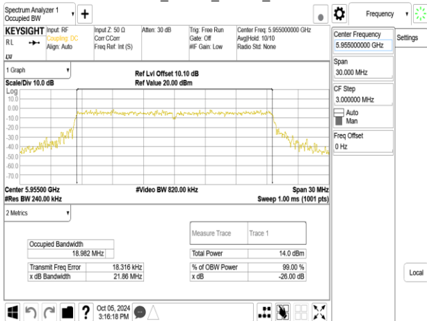
802.11be_20MHz_Chain0_5955MHz
