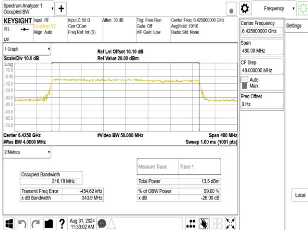
802.11be_320MHz_Chain0_6425MHz
