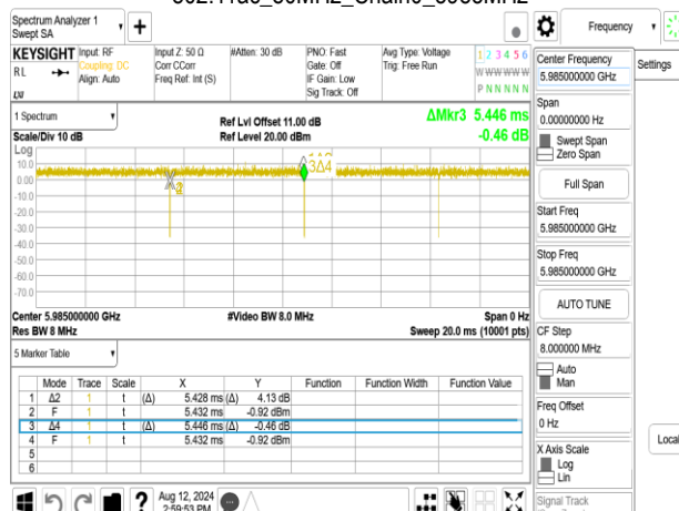
802.11ac_80MHz_Chain0_5985MHz
