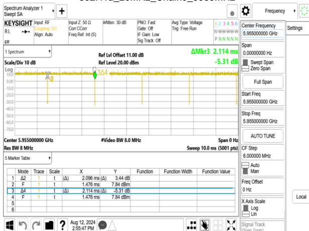
802.11n_20MHz_Chain0_5955MHz
