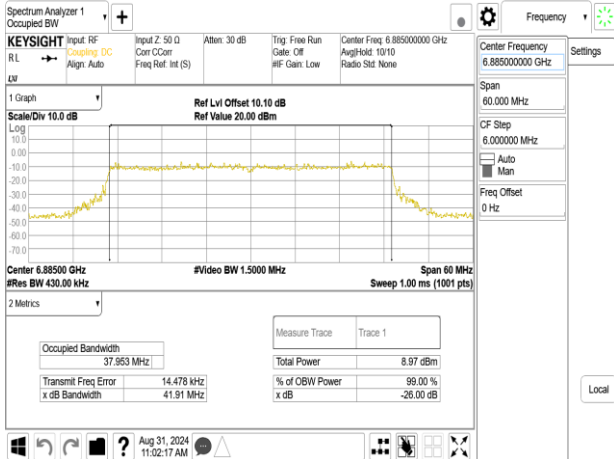
802.11be_40MHz_Chain1_6885MHz
