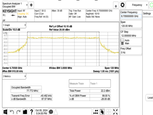
802.11be_80MHz_Chain1_6705MHz
