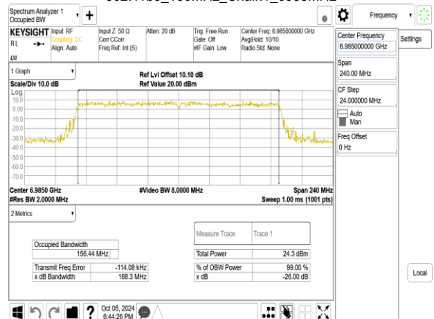
802.11be_160MHz_Chain1_6985MHz
