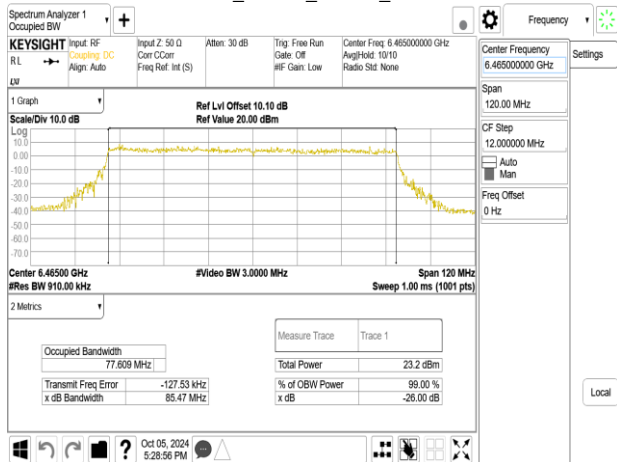
802.11be_80MHz_Chain1_6465MHz
