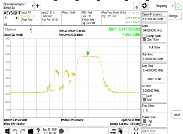
802.11be_20MHz_Chain1_6415MHz_RU106_54
