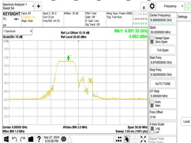
802.11be_20MHz_Chain0_6895MHz_52+26_MRU1
