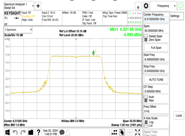
802.11be_20MHz_Chain0_6515MHz_106+26_MRU2
