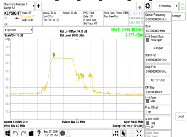
802.11be_20MHz_Chain1_5955MHz_RU26_0
