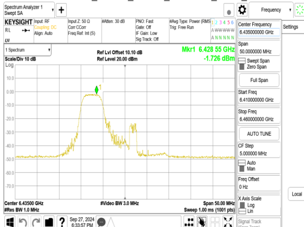
802.11be_20MHz_Chain0_6435MHz_RU52_37
