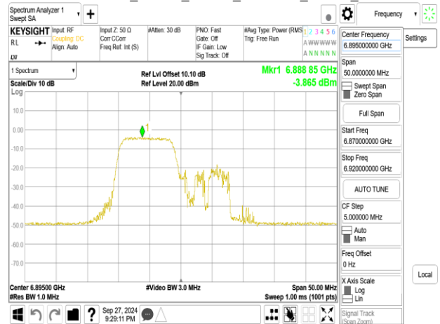
802.11be_20MHz_Chain0_6895MHz_RU26_0
