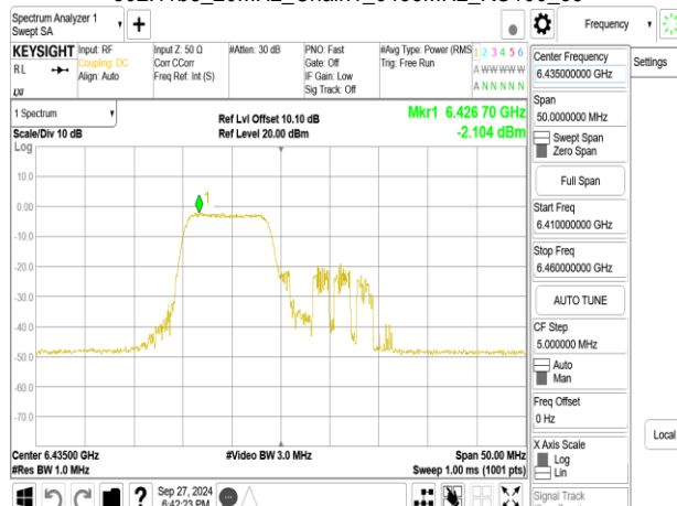
802.11be_20MHz_Chain1_6435MHz_RU106_53
