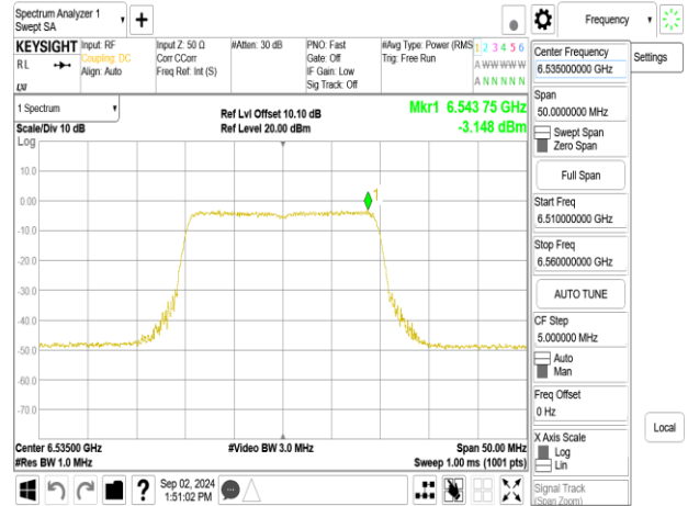
802.11be_20MHz_Chain0_6535MHz_106+26_MRU1
