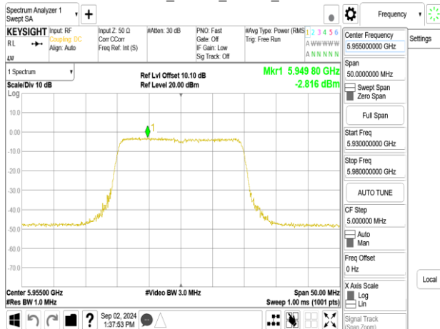
802.11be_20MHz_Chain1_5955MHz_106+26_MRUI
