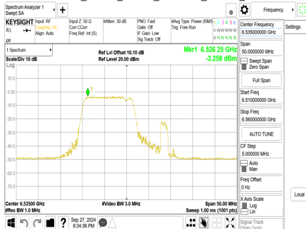
802.11be_20MHz_Chain1_6535MHz_52+26_MRU1
