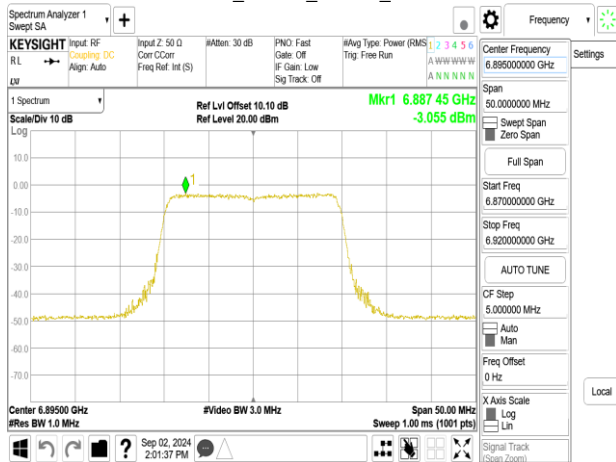
802.11be_20MHz_Chain0_6895MHz_106+26_MRU1
