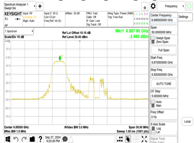
802.11be_20MHz_Chain0_6895MHz_RU52_37
