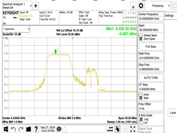
802.11be_20MHz_Chain0_6435MHz_RU26_0
