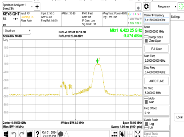
802.11be_20MHz_Chain1_6415MHz_RU52_40
