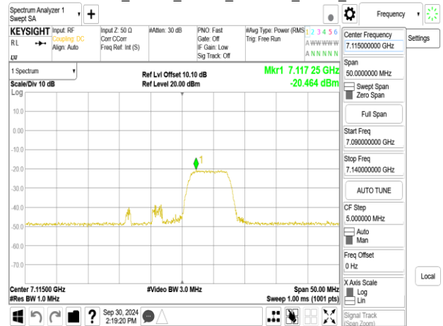
802.11be_20MHz_Chain0_7115MHz_RU106_54
