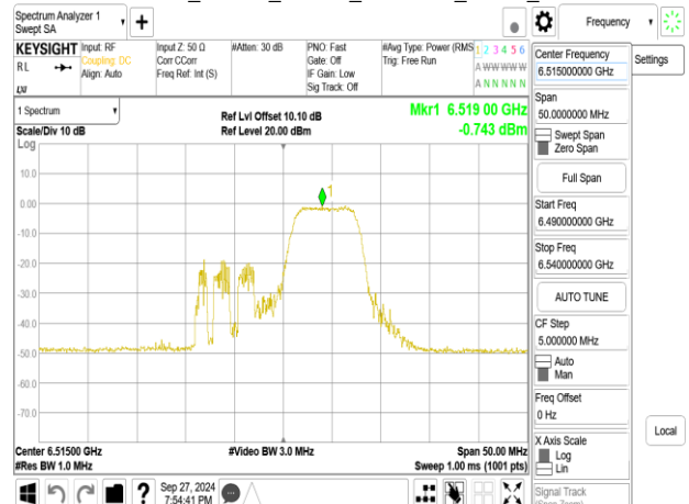
802.11be_20MHz_Chain1_6515MHz_52+26_MRU3
