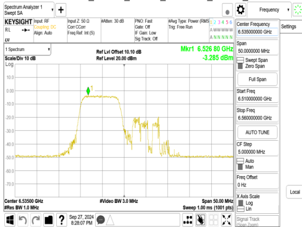
802.11be_20MHz_Chain0_6535MHz_RU26_0
