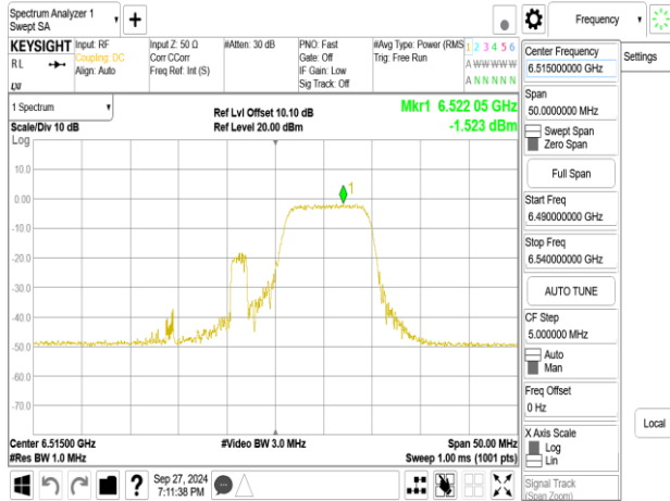
802.11be_20MHz_Chain0_6515MHz_RU26_8
