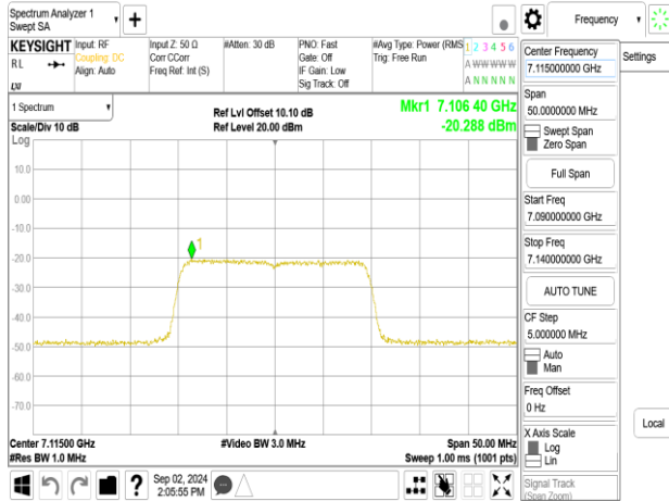
802.11be_20MHz_Chain0_7115MHz_106+26_MRUI2
