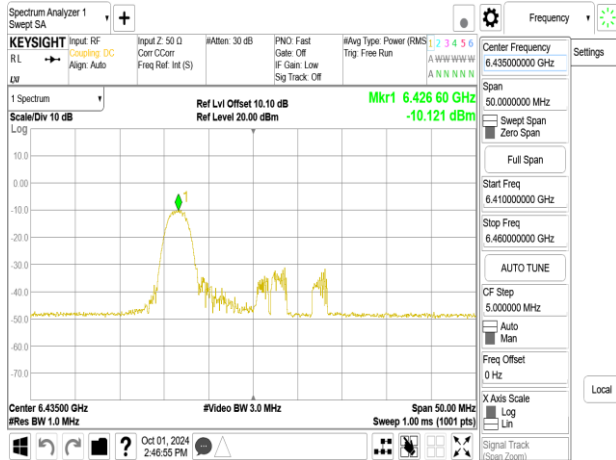
802.11be_20MHz_Chain1_6435MHz_RU52_37
