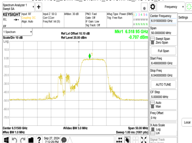
802.11be_20MHz_Chain1_6515MHz_RU26_8
