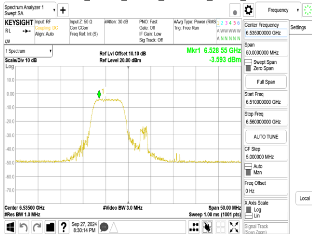
802.11be_20MHz_Chain0_6535MHz_RU106_53
