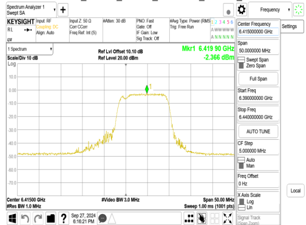
802.11be_20MHz_Chain1_6415MHz_52+26_MRU3
