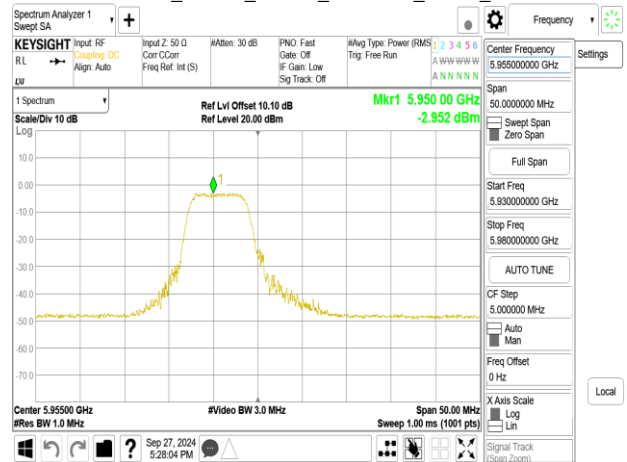
802.11be_20MHz_Chain1_5955MHz_RU106_53
