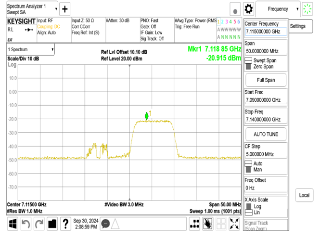
802.11be_20MHz_Chain0_7115MHz_RU26_8
