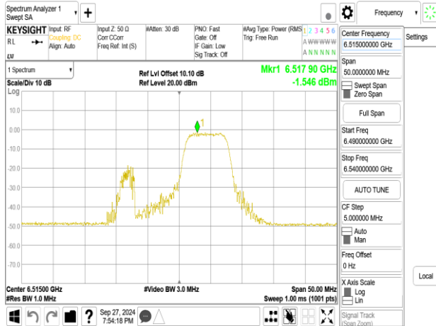
802.11be_20MHz_Chain0_6515MHz_RU106_54
