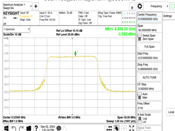
802.11be_20MHz_Chain1_6535MHz_106+26_MRU1
