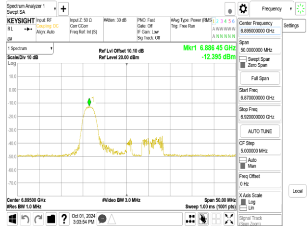
802.11be_20MHz_Chain0_6895MHz_RU52_37
