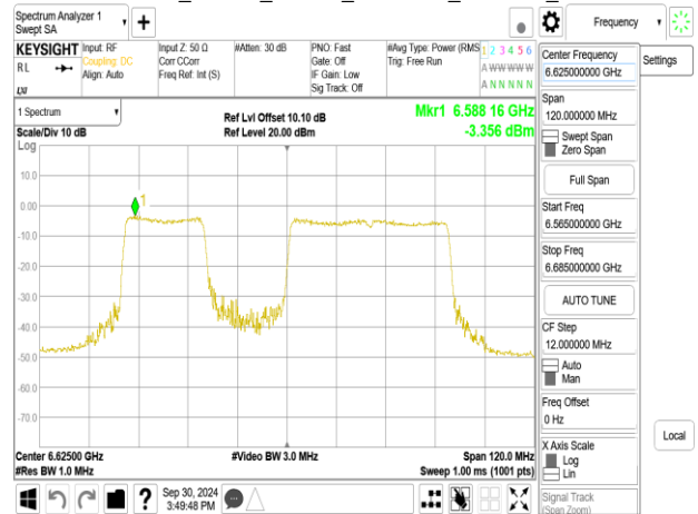
802.11be_80MHz_Chain1_6625MHz_RU484_65
