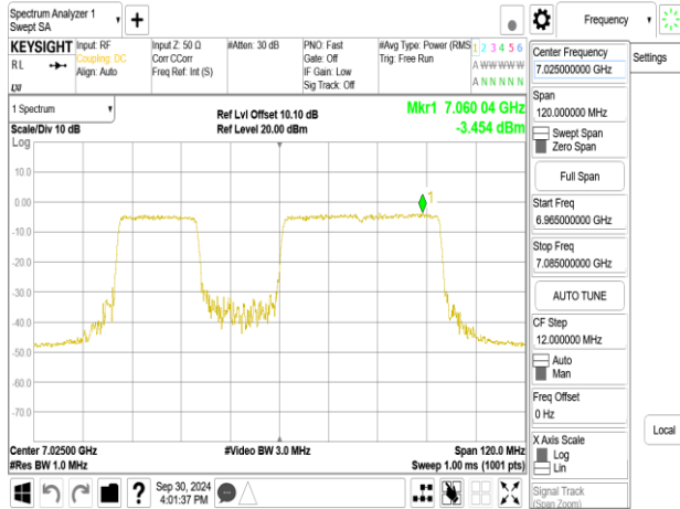
802.11be_80MHz_Chain0_7025MHz_RU484_66
