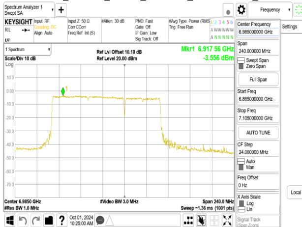
802.11be_160MHz_Chain0_6985MHz_996+484_MRU2
