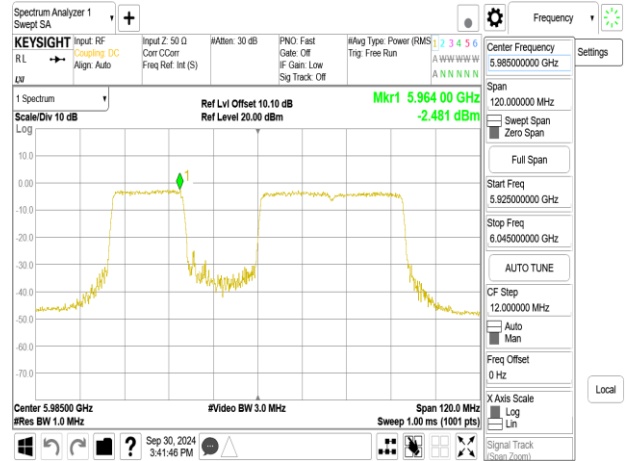
802.11be_80MHz_Chain1_5985MHz_RU484_65
