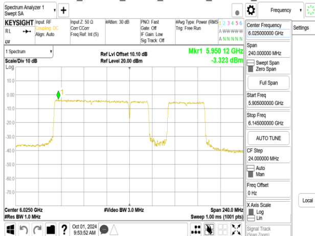
802.11be_160MHz_Chain0_6025MHz_996+484_MRU4
