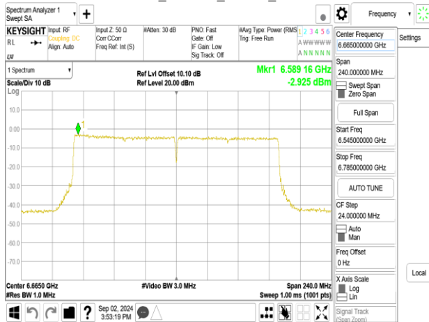
802.11be_160MHz_Chain0_6665MHz_996+484+242_MRU2
