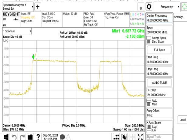
802.11be_160MHz_Chain0_6665MHz_996+484+242_MRU4
