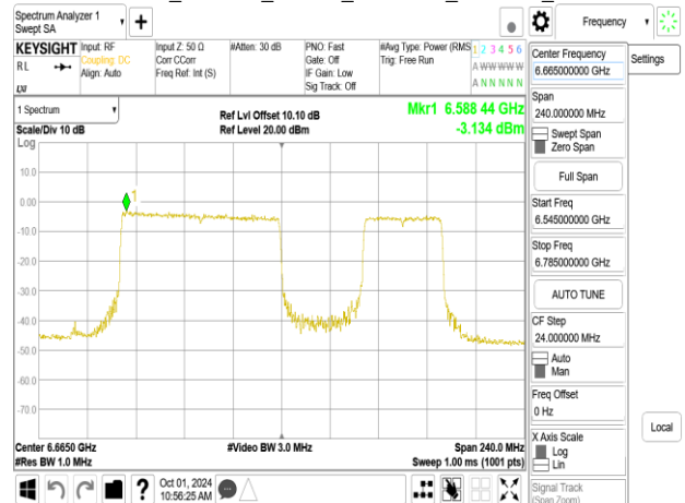
802.11be_160MHz_Chain0_6665MHz_996+484_MRU4
