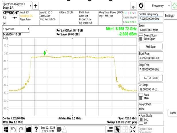
802.11be_80MHz_Chain1_7025MHz_484+242_MR1
