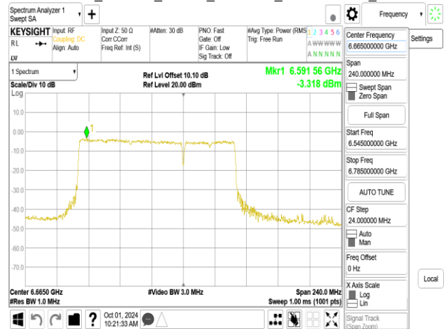
802.11be_160MHz_Chain0_6665MHz_996+484_MRU2
