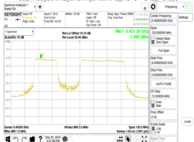
802.11be_80MHz_Chain1_6465MHz_RU484+242_Punc20
