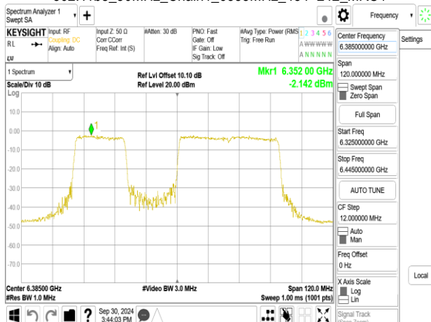
802.11be_80MHz_Chain1_6385MHz_484+242_MRU1
