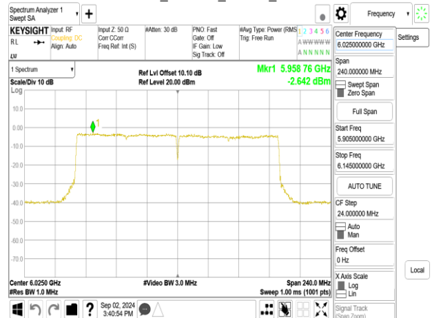
802.11be_160MHz_Chain1_6025MHz
