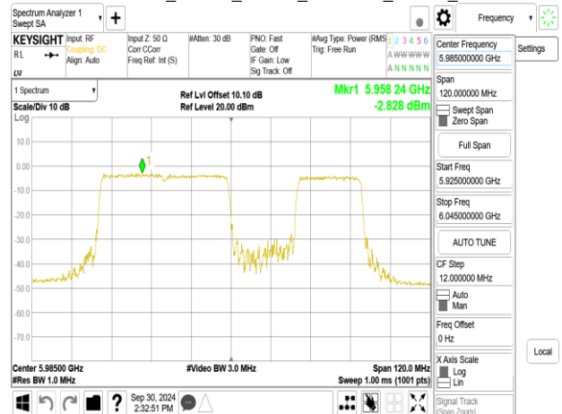
802.11be_80MHz_Chain1_5985MHz_RU484_65
