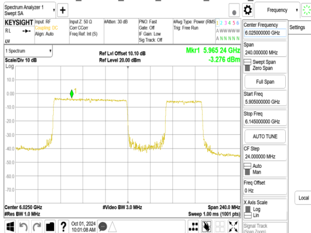
802.11be_160MHz_Chain0_6025MHz_996+484_MRU4
