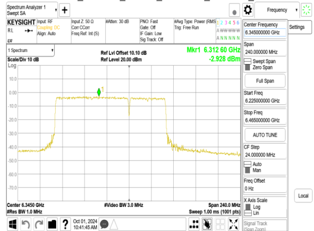
802.11be_160MHz_Chain0_6345MHz_RU996_S67
