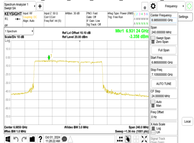
802.11be_160MHz_Chain0_6985MHz_996+484+242_MRU4
