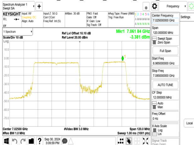
802.11be_80MHz_Chain0_7025MHz_RU484_66
