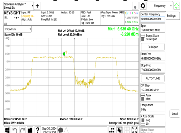
802.11be_80MHz_Chain0_6945MHz_RU484_65
