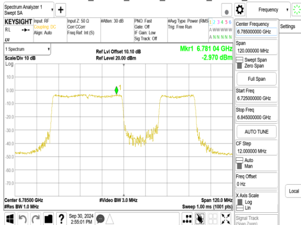
802.11be_80MHz_Chain1_6785MHz_RU484_66
