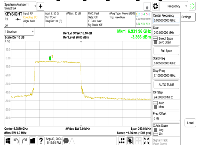
802.11be_160MHz_Chain0_6985MHz_RU996_S67
