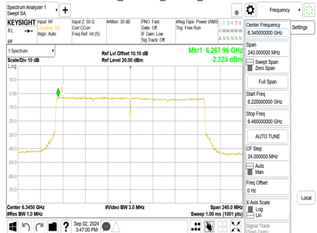
802.11be_160MHz_Chain0_6345MHz
