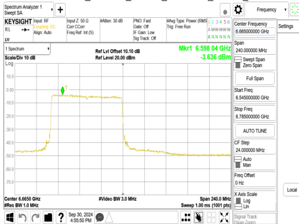
802.11be_160MHz_Chain0_6665MHz_RU996_S67
