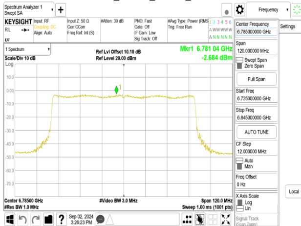
802.11be_80MHz_Chain1_6785MHz_484+242_MRU1
