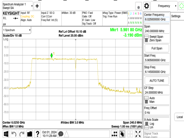
802.11be_160MHz_Chain0_6025MHz_996+484_MRU2
