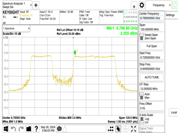
802.11be_80MHz_Chain1_6785MHz_RU484_66
