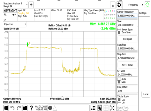
802.11be_160MHz_Chain1_6665MHz_996+484_MRU2
