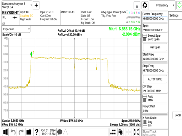
802.11be_160MHz_Chain1_6665MHz_RU996_67
