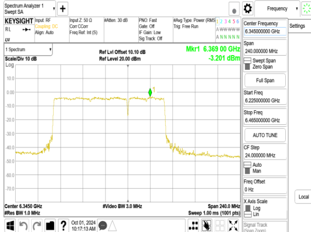
802.11be_160MHz_Chain1_6345MHz_996+484+242_MRU5
