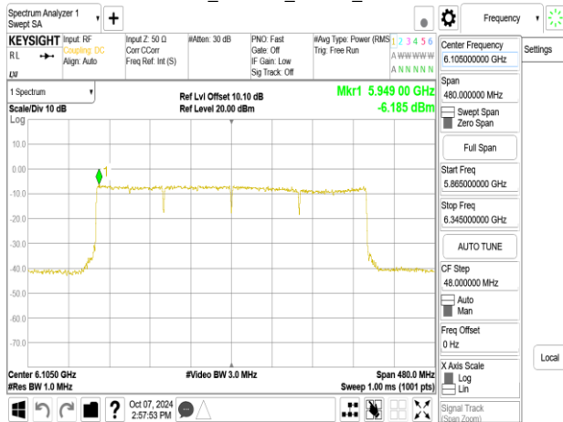
802.11be_320MHz_Chain0_6105MHz_2x996+484_MRUA
