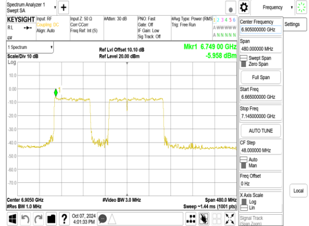
802.11be_320MHz_Chain1_6905MHz_RU996x2+484_Punc40
