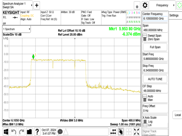
802.11be_320MHz_Chain0_6105MHz_3x996+484_MRUA
