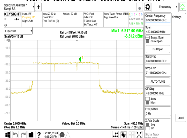
802.11be_320MHz_Chain0_6905MHz_RU996x2+484_Punc40
