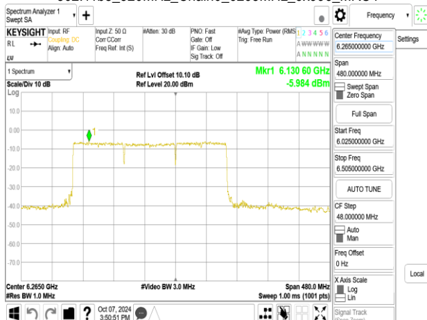
802.11be_320MHz_Chain0_6265MHz_3x996_MRU4
