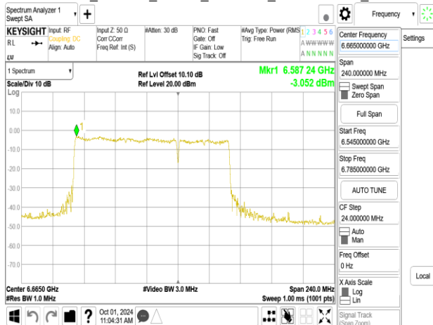
802.11be_160MHz_Chain1_6665MHz_996+484+242_MRU2
