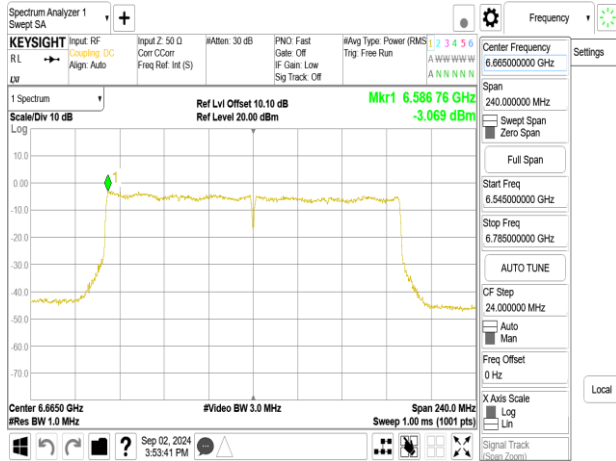
802.11be_160MHz_Chain1_6665MHz_996+484+242_MRU2
