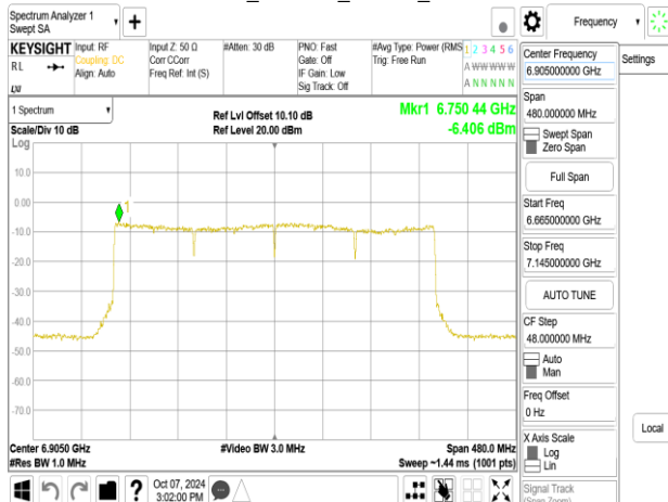
802.11be_320MHz_Chain0_6905MHz_2x996+484_MRU6
