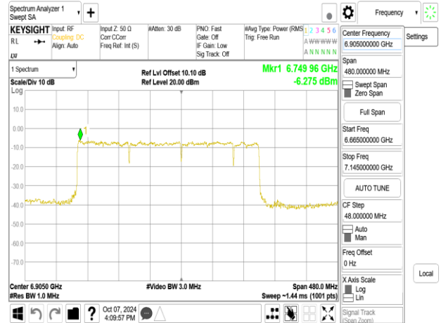
802.11be_320MHz_Chain1_6905MHz_3x996+484 MRU1
