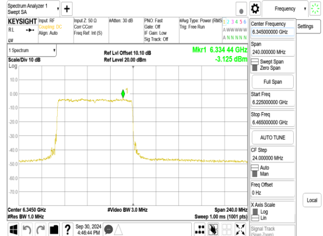
802.11be_160MHz_Chain1_6345MHz_RU996_S67
