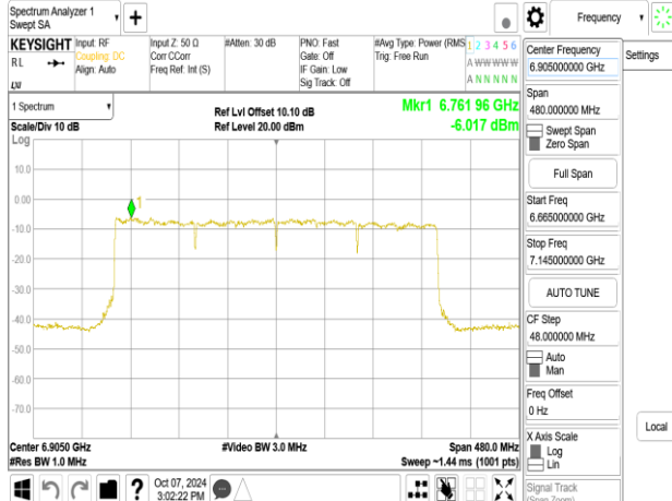
802.11be_320MHz_Chain1_6905MHz_2x996+484 MRU6
