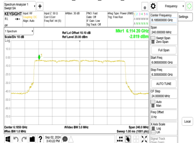
802.11be_160MHz_Chain1_6185MHz
