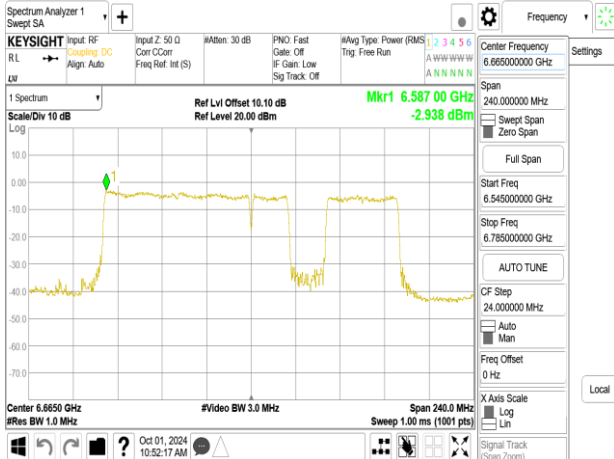
802.11be_160MHz_Chain1_6665MHz_RU996_S67
