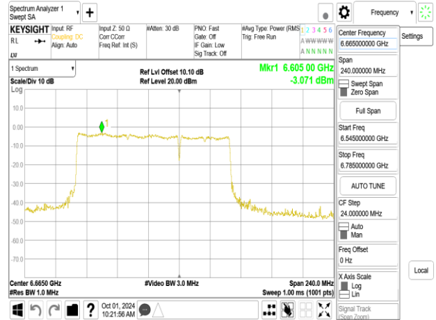
802.11be_160MHz_Chain1_6665MHz_996+484_MRU2
