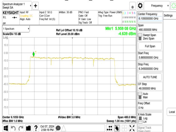
802.11be_320MHz_Chain1_6105MHz_2x996+484_MRUA
