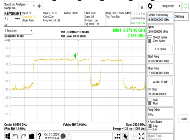
802.11be_160MHz_Chain1_6985MHz_RU996_S67
