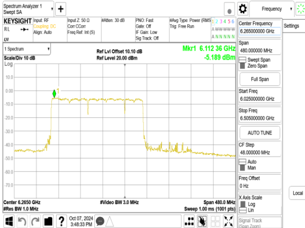
802.11be_320MHz_Chain1_6265MHz_3x996+484_MRUE
