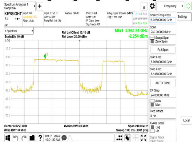
802.11be_160MHz_Chain1_6025MHz_RU996_67
