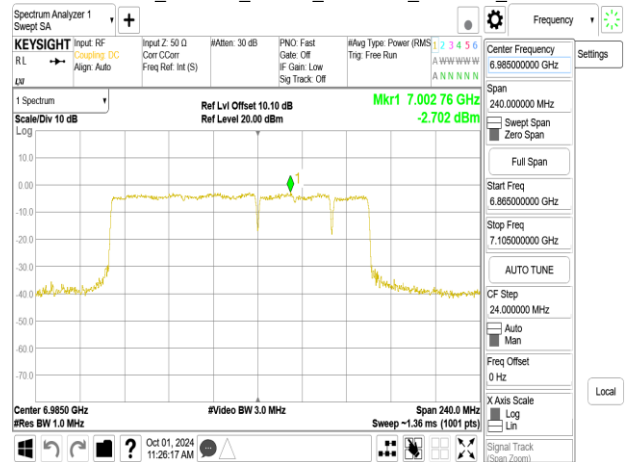
802.11be_160MHz_Chain1_6985MHz_RU996_67
