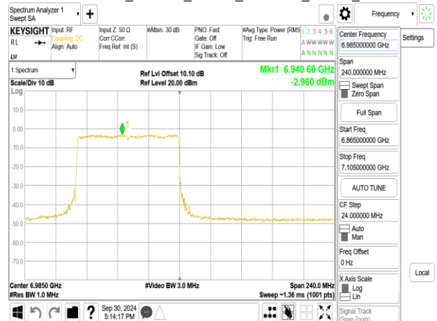
802.11be_160MHz_Chain1_6985MHz_RU996_S67
