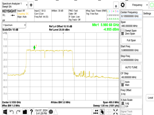
802.11be_320MHz_Chain1_6105MHz_3x996+484_MRUA
