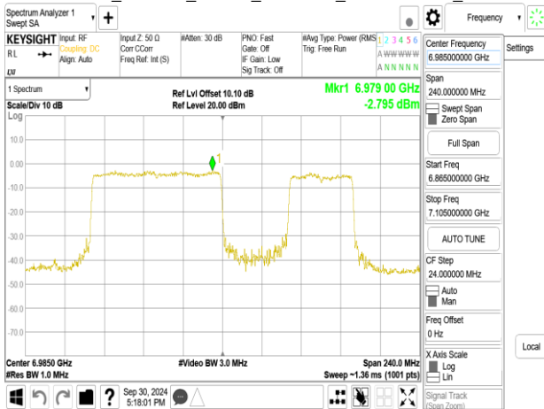
802.11be_160MHz_Chain1_6985MHz_996+484+242_MR48
