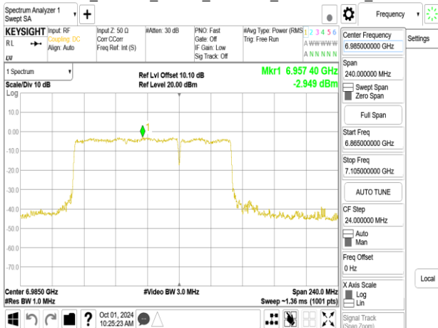
802.11be_160MHz_Chain1_6985MHz_996+484_MR42
