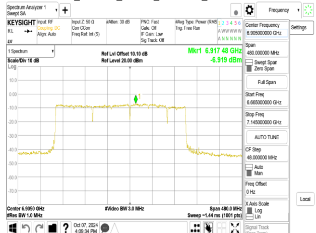
802.11be_320MHz_Chain0_6905MHz_3x996_MRU4
