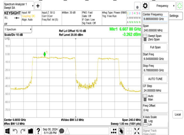
802.11be_160MHz_Chain1_6665MHz_996+484+242_MRU8
