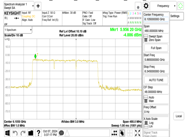
802.11be_320MHz_Chain1_6105MHz_RU996x2+484_Punc40
