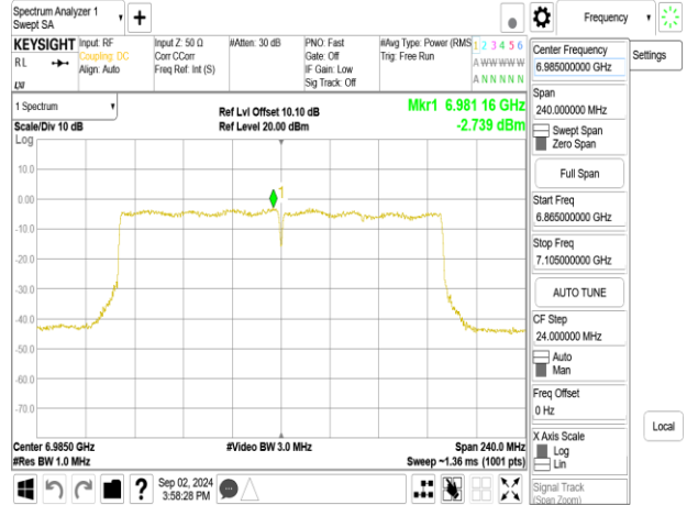
802.11be_160MHz_Chain1_6985MHz_996+484+242_MRUI2
