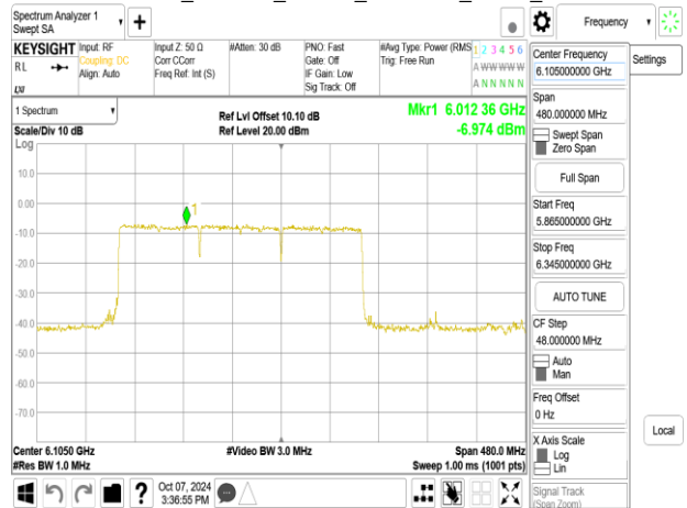
802.11be_320MHz_Chain0_6105MHz_RU996x2+484_Punc40
