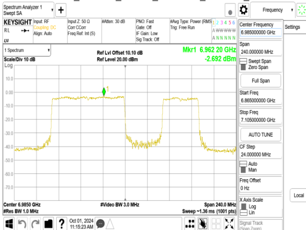
802.11be_160MHz_Chain1_6985MHz_996+484_MR42
