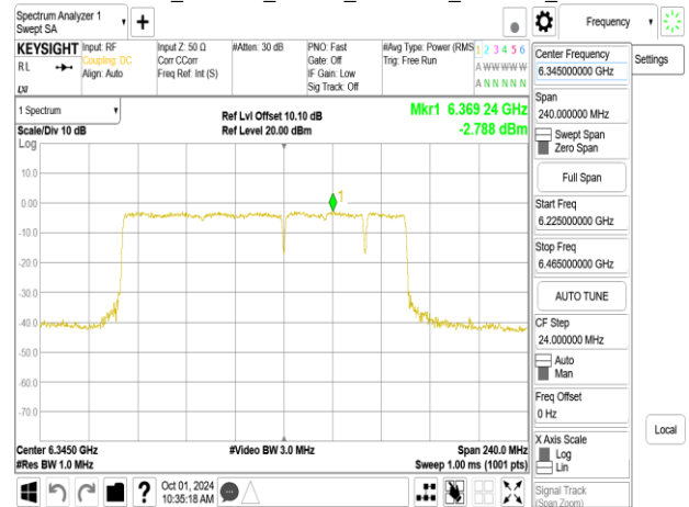
802.11be_160MHz_Chain1_6345MHz_996+484_MRU3
