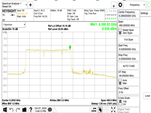
802.11be_320MHz_Chain0_6265MHz_3x996+484_MRU8
