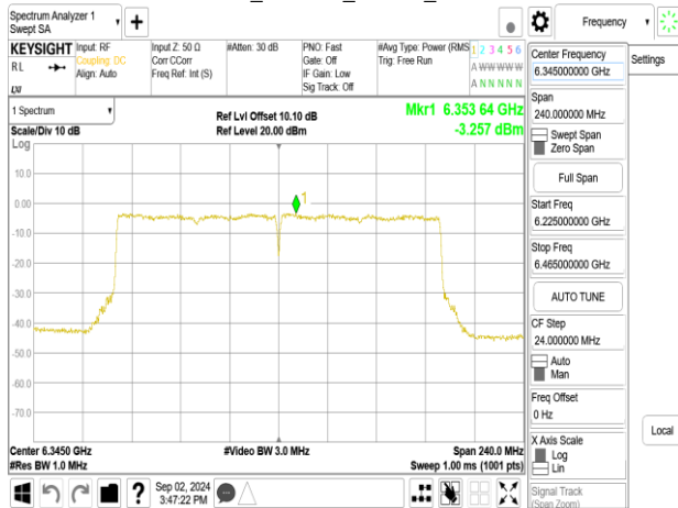
802.11be_160MHz_Chain1_6345MHz_996+484+242_MRU1
