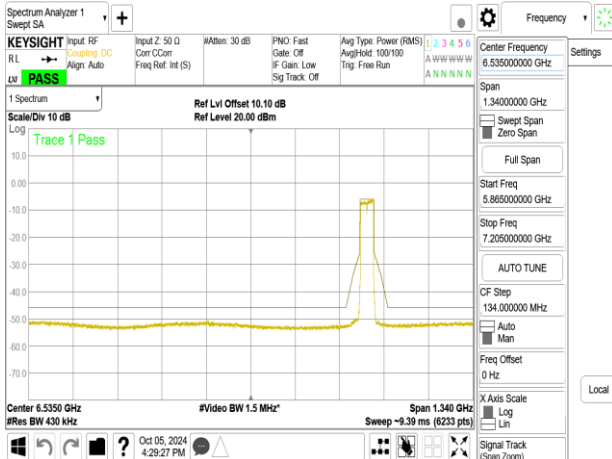
802.11be_40MHz_Chain0_6925MHz
