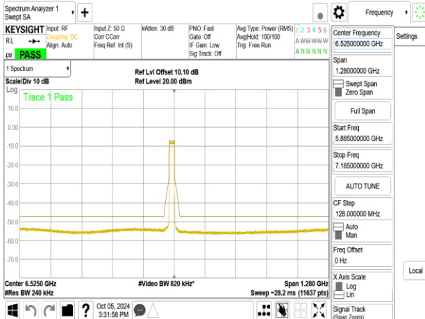
802.11be_20MHz_Chain0_6535MHz
