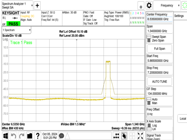
802.11be_40MHz_Chain0_6885MHz
