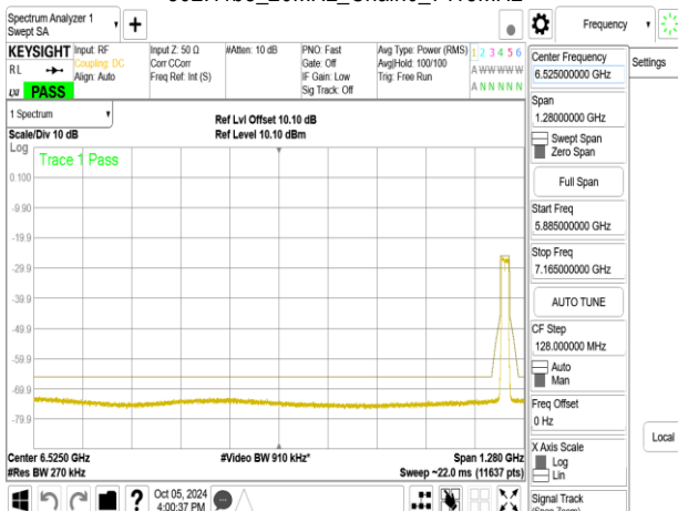
802.11be_20MHz_Chain0_7115MHz
