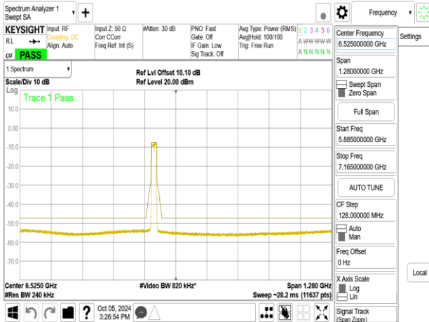
802.11be_20MHz_Chain1_6475MHz
