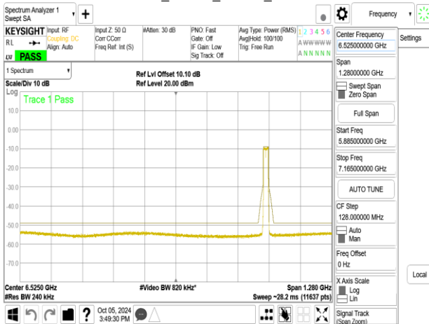
802.11be_20MHz_Chain0_6995MHz
