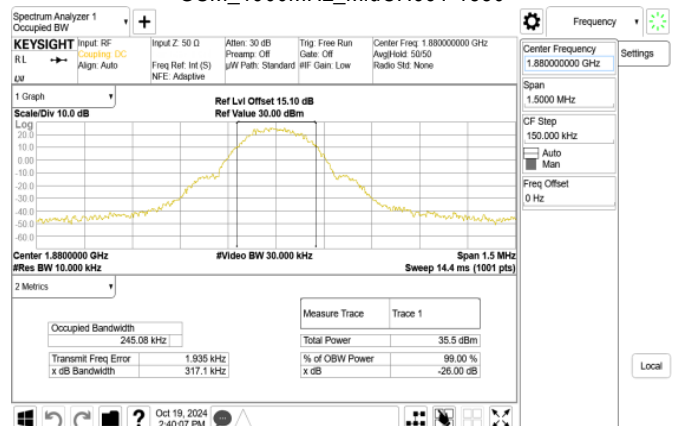
GSM_1900MHz_MidCH661-1880
