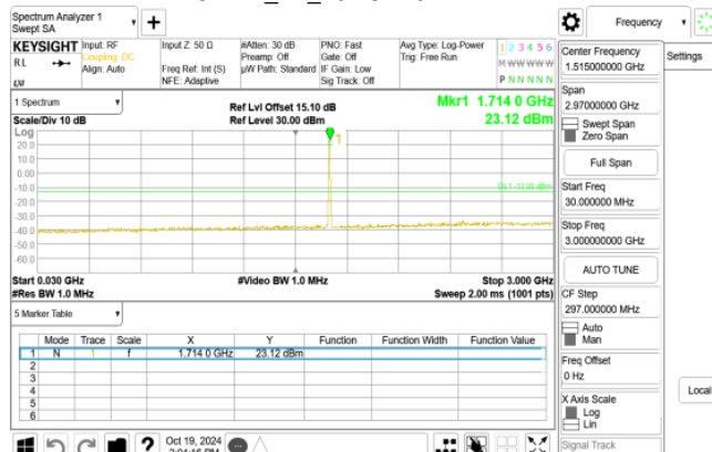
WCDMA_B4_LowCH1312-1712.4
