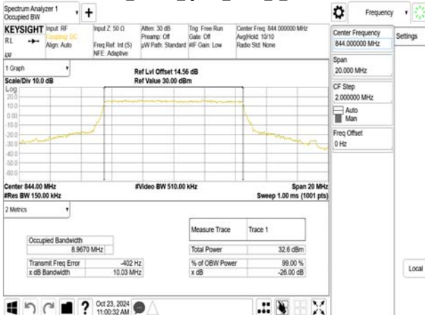
Band5_10MHz_QPSK_RB50_0_CH20600
