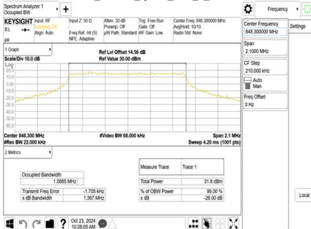
Band5 1.4MHz QPSK_RB6_0_CH20643
