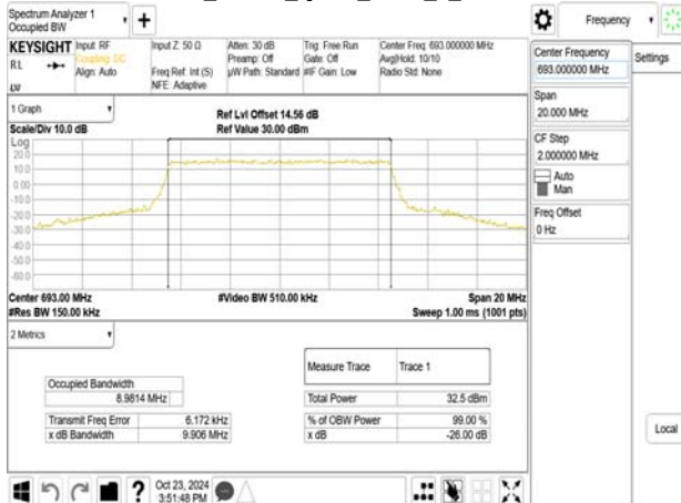
Band71_10MHz_QPSK_RB50_0_CH133422
