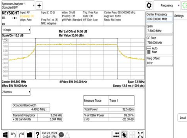
Band71_5MHz_QPSK_RB25_0_CH133447
