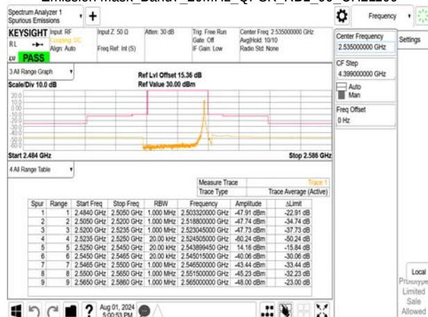
Emission Mask_Band7_20MHz_QPSK_RB1_99_CH21100
