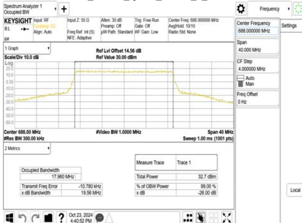
Band71_20MHz_QPSK_RB100_0_CH133372
