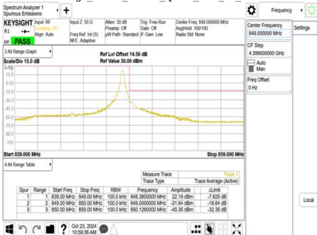
Band Edge_Band5_10MHz_QPSK_RB50_0_CH20450
