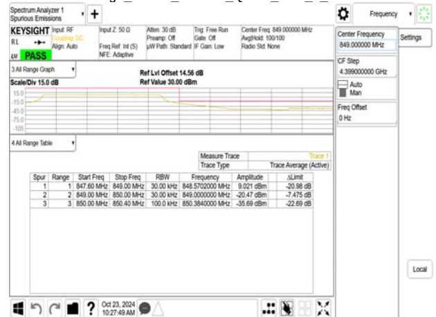
Band Edge_Band5_3MHz_QPSK_RB1_0_CH20415
