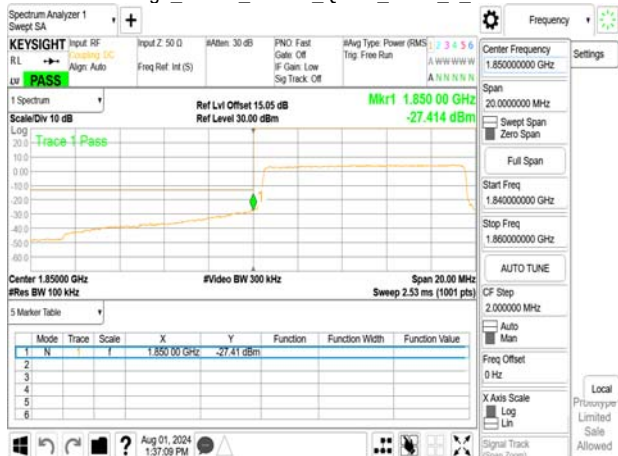
Band Edge_Band2_10MHz_QPSK_RB50_0_CH18650
