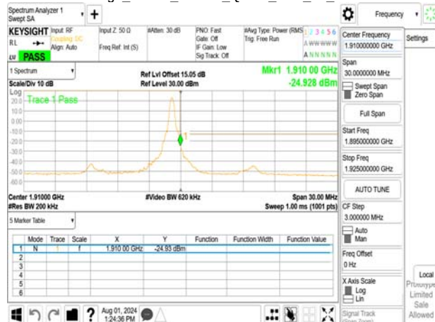
Band Edge_Band2_15MHz_QPSK_RB1_74_CH19125
