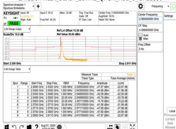
Emission Mask_Band7_20MHz_QPSK_RB1_99_CH20850
