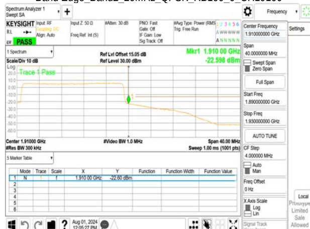
Band Edge_Band2_20MHz_QPSK_RB100_0_CH19100
