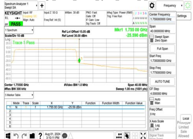
Band Edge_Band4_20MHz_QPSK_RB100_0_CH20300
