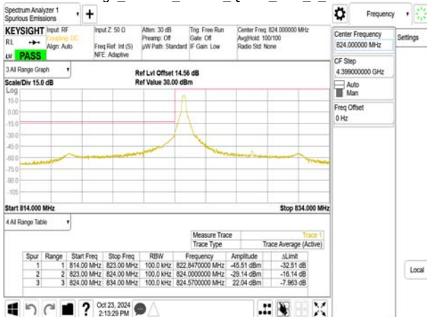
Band Edge_Band26_10MHz_QPSK_RB1_49_CH26990
