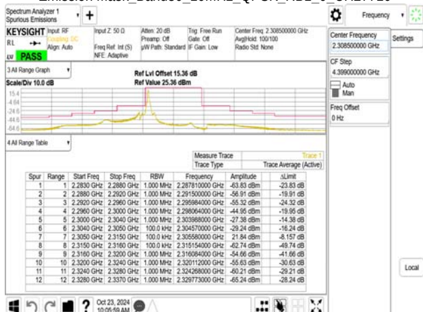
Emission Mask_Band30_10MHz_QPSK_RB1_49_CH27710
