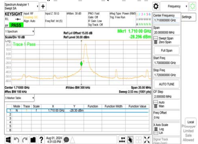
Band Edge_Band66_10MHz_QPSK_RB1_49_CH132622
