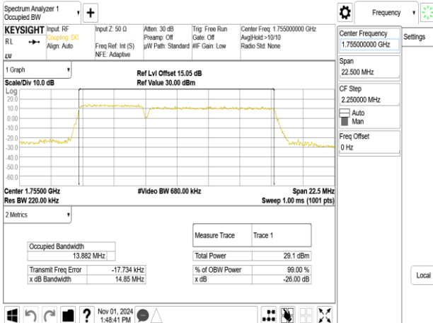
Band66B_10MHz+5MHz_QPSK_RB50-0+RB25-0_CH132397+CH132469
