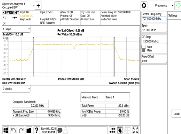
Band12B_5MHz+10MHz_QPSK_RB25-0+RB50-0_CH23048+CH23120
