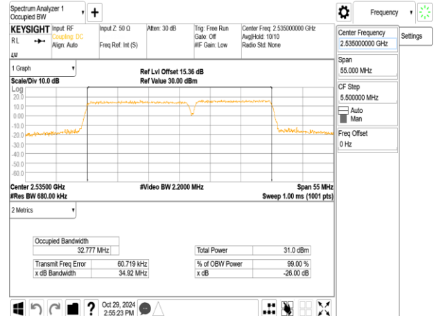
Band7_20MHz+15MHz_64QAM_RB100-0+RB75-0_CH21026+CH21197
