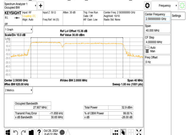
Band41_10MHz+20MHz_QPSK_RB50-0+RB100-0_CH40526+CH40670
