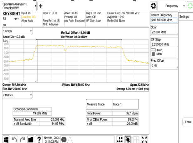
Band12B_5MHz+10MHz_QPSK_RB25-0+RB50-0_CH23048+CH23120
