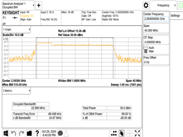
Band41_20MHz+5MHz_QPSK_RB100-0+RB25-0_CH40595+CH40712
