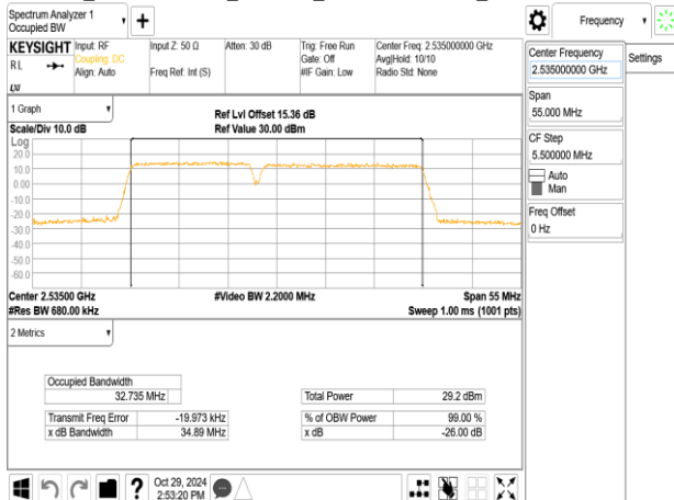
Band7_20MHz+15MHz_QPSK_RB100-0+RB75-0_CH21026+CH21197
