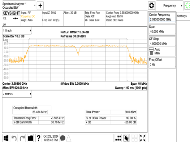
Band41_20MHz+10MHz_QPSK_RB100-0+RB50-0_CH40571+CH40715
