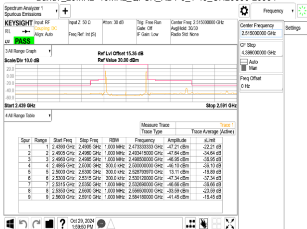
Band7_20MHz+10MHz_QPSK_RB1-0_1-49_CH21051-21195
