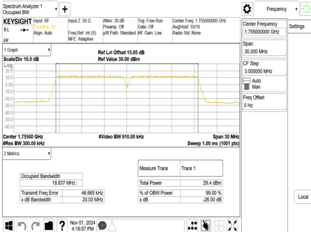
Band66B_15MHz+5MHz_QPSK_RB75-0+RB25-0_CH132398+CH132491
