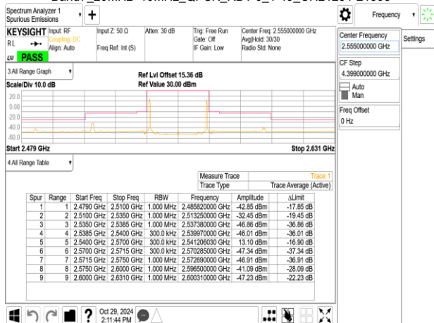
Band7_20MHz+10MHz_QPSK_RB1-0_1-49_CH21251-21395
