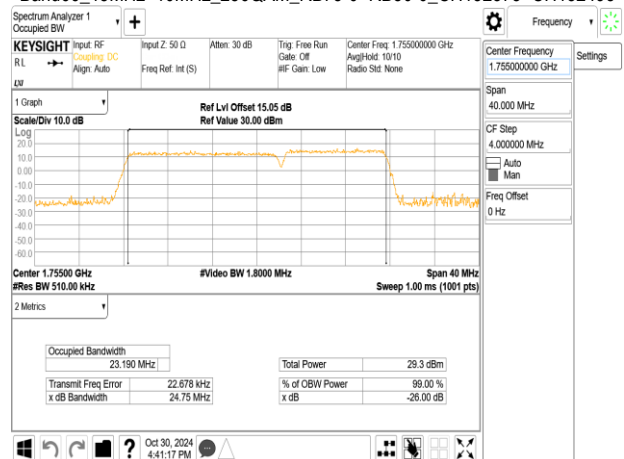
Band66_20MHz+5MHz_QPSK_RB100-0+RB25-0_CH132397+CH132514
