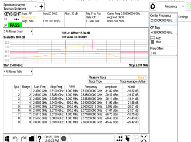
Band7_20MHz+10MHz_QPSK_RB100-0_50-0_CH21251-21395
