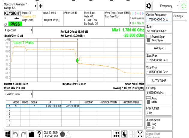
Band66 20MHz+20MHz_QPSK_RB1-0_1-0_CH132072-132270
