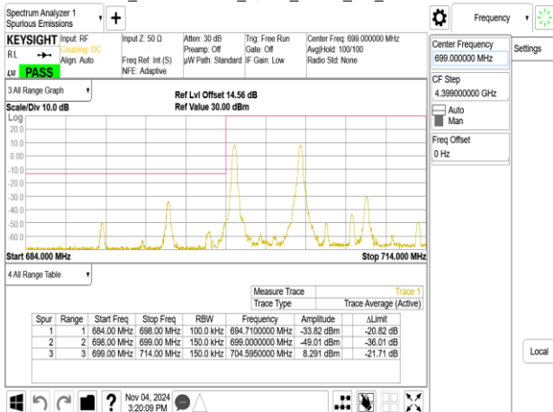
Band12B_5MHz+10MHz_QPSK_RB1-24_1-49_CH23058-23130
