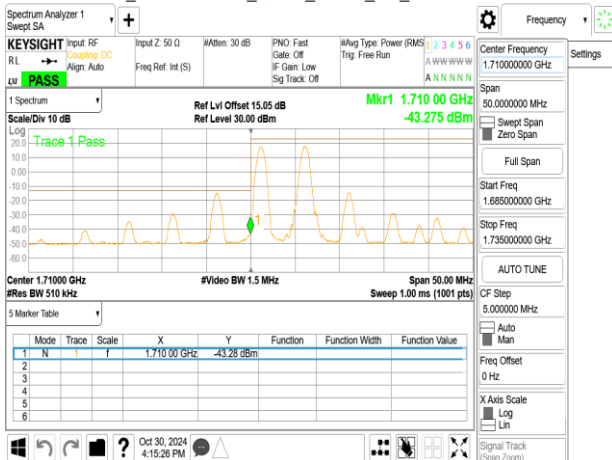
Band66 5MHz+20MHz_QPSK_RB1-25_1-99_CH132455-132572
