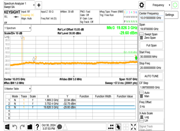
Band2_20MHz+20MHz_QPSK_RB1-99_1-0_CH18801-18999
