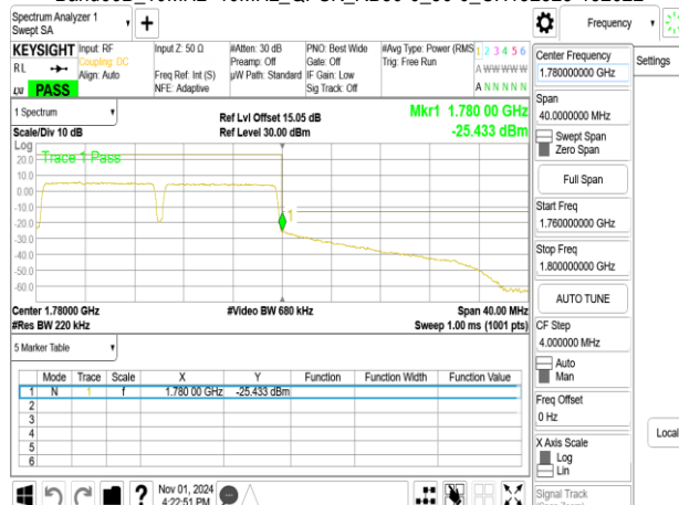
Band66B_10MHz+10MHz_QPSK_RB50-0_50-0_CH132523-132622
