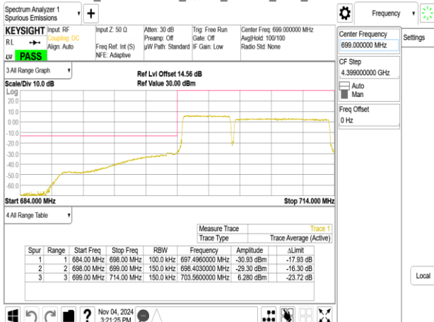
Band12B_5MHz+10MHz_QPSK_RB25-0_50-0_CH23038-23110
