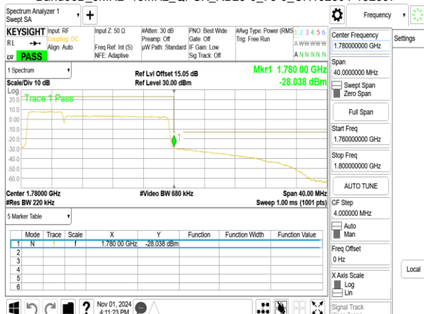
Band66B_10MHz+10MHz_QPSK_RB1-0_1-0_CH132022-132121
