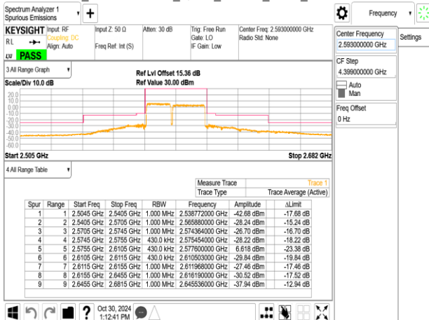
Band41_15MHz+20MHz_QPSK_RB75-0_100-0_CH40523-40694
