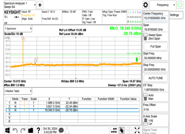
Band2_20MHz+20MHz_QPSK_RB1-99_1-0_CH18902-19100
