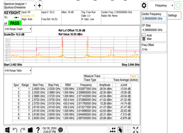
Band41_20MHz+20MHz_QPSK_RB1-0_1-99_CH40521-40719
