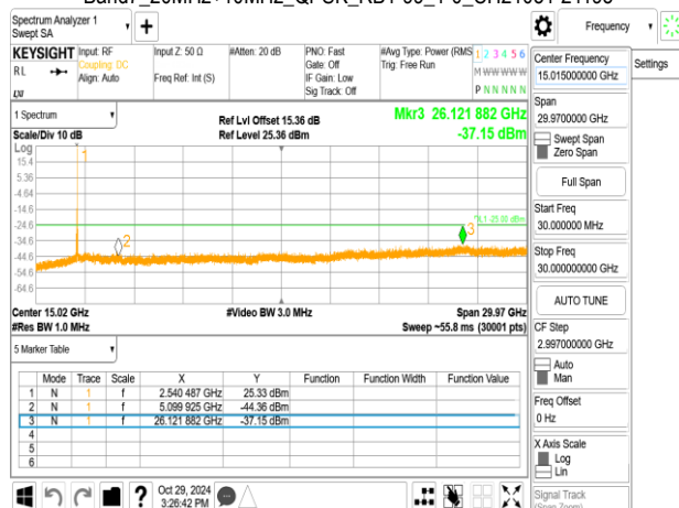
Band7_20MHz+10MHz_QPSK_RB1-99_1-0_CH21251-21395
