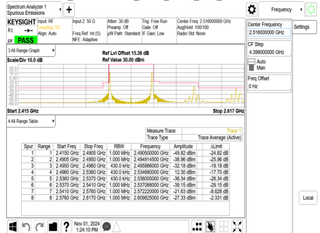
Band41_20MHz+20MHz_QPSK_RB1-0_1-99_CH40521-40719
