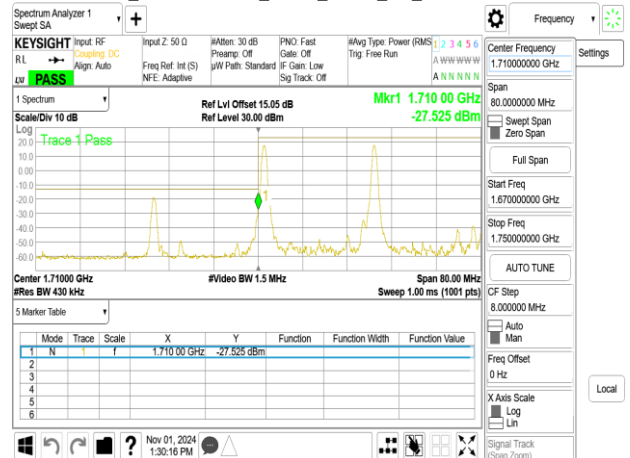
Band66 20MHz+20MHz_QPSK_RB1-99_1-99_CH132374-132572
