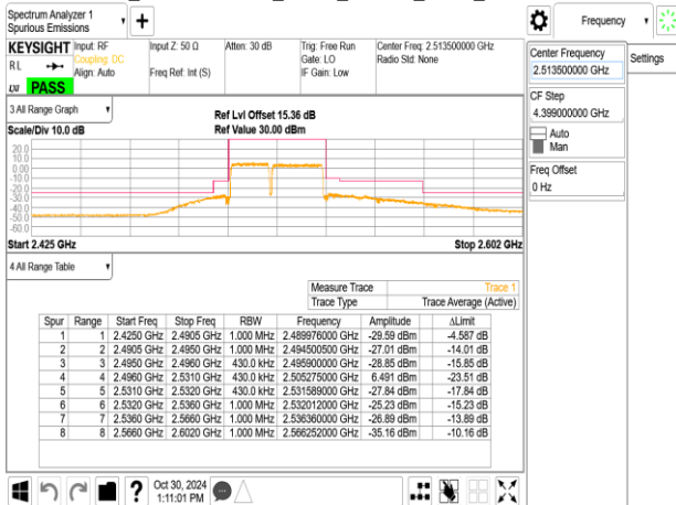
Band41_15MHz+20MHz_QPSK_RB75-0_100-0_CH40523-40694
