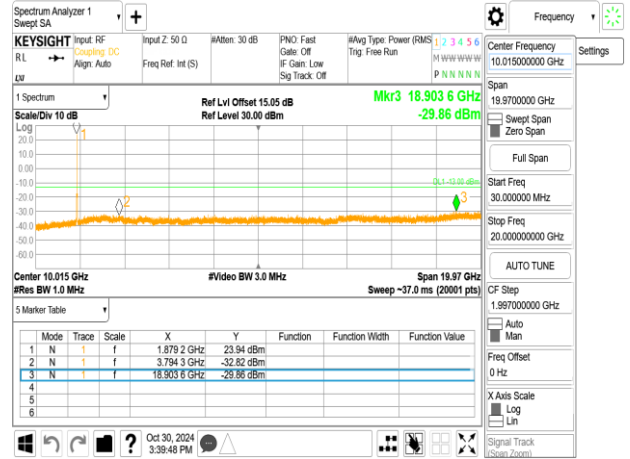
Band2_20MHz+20MHz_QPSK_RB1-99_1-0_CH18902-19100
