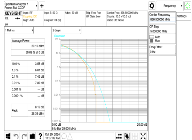
Band5_10MHz+5MHz_256QAM_RB50-0+RB25-0_CH20500+CH20572
