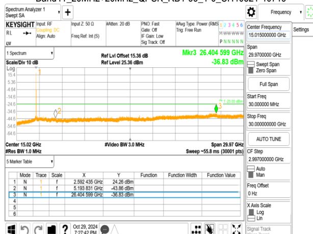
Band41_20MHz+20MHz_QPSK_RB1-99_1-0_CH41292-41490
