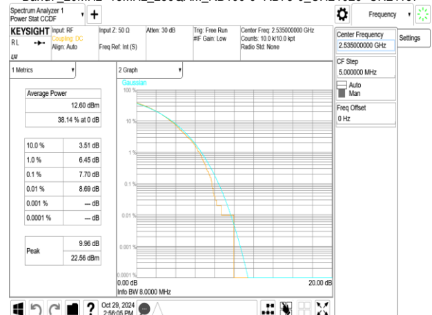
Band7_20MHz+15MHz_256QAM_RB100-0+RB75-0_CH21026+CH21197
