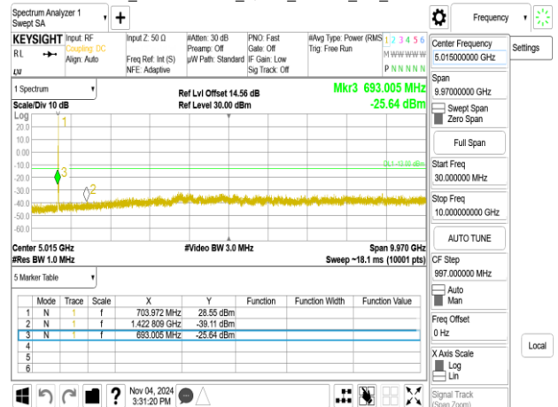
Band12B_5MHz+10MHz_QPSK_RB1-24_1-0_CH23048-23120
