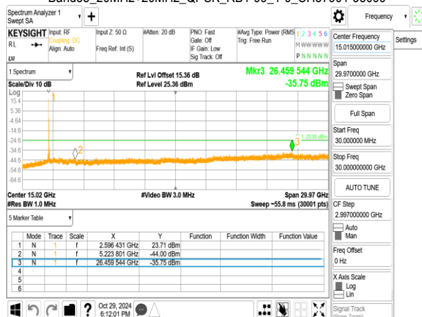
Band38_20MHz+20MHz_QPSK_RB1-99_1-0_CH37952-38150
