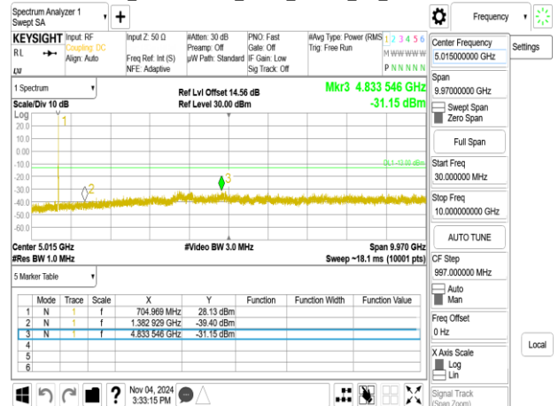
Band12B_5MHz+10MHz_QPSK_RB1-24_1-0_CH23058-23130
