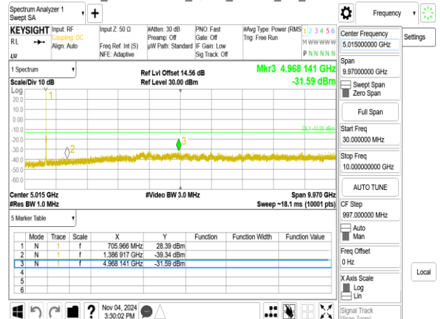
Band12B_5MHz+10MHz_QPSK_RB1-24_1-0_CH23058-23130
