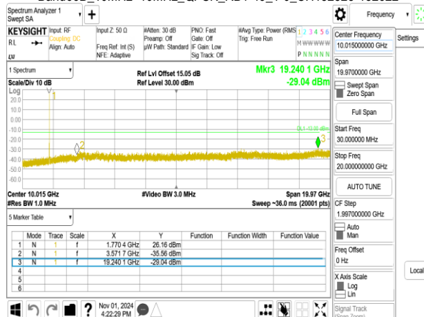
Band66B_10MHz+10MHz_QPSK_RB1-49_1-0_CH132523-132622
