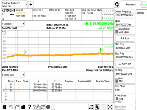
Band7_20MHz+20MHz_QPSK_RB1-99_1-0_CH21152-21350
