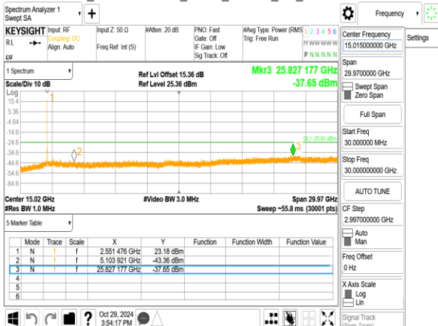
Band7_20MHz+20MHz_QPSK_RB1-99_1-0_CH21152-21350
