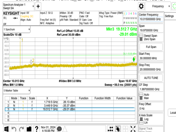
Band66B_10MHz+10MHz_QPSK_RB1-49_1-0_CH132373-132472
