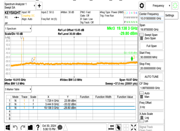
Band66_20MHz+20MHz_QPSK_RB1-99_1-0_CH132323-132521
