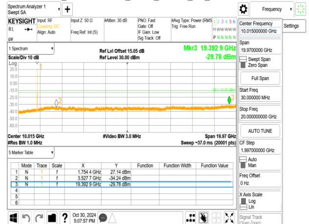
Band66_20MHz+20MHz_QPSK_RB1-99_1-0_CH132374-132572
