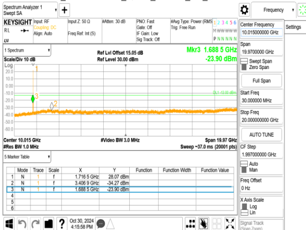
Band66_5MHz+20MHz_QPSK_RB1-24_1-0_CH132303-132447
