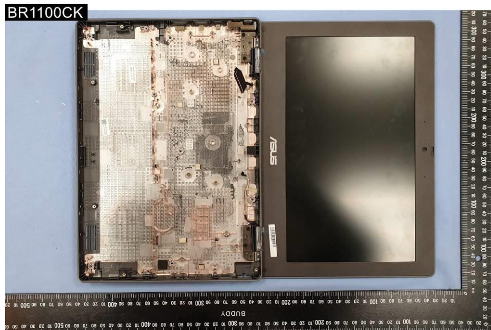
EUT Photo (14)
