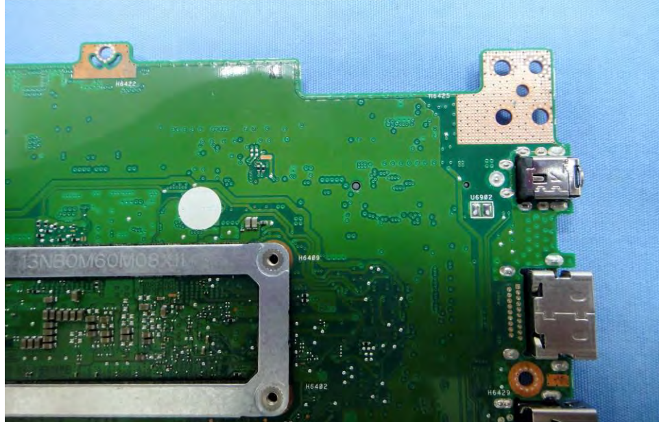
EUT Photo (50)
