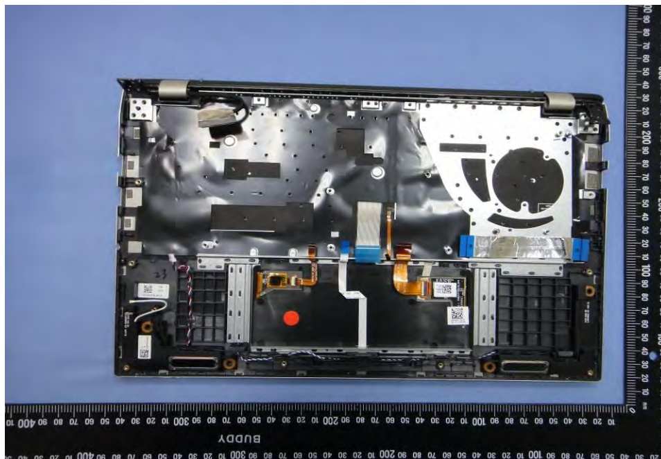
EUT Photo (60)
