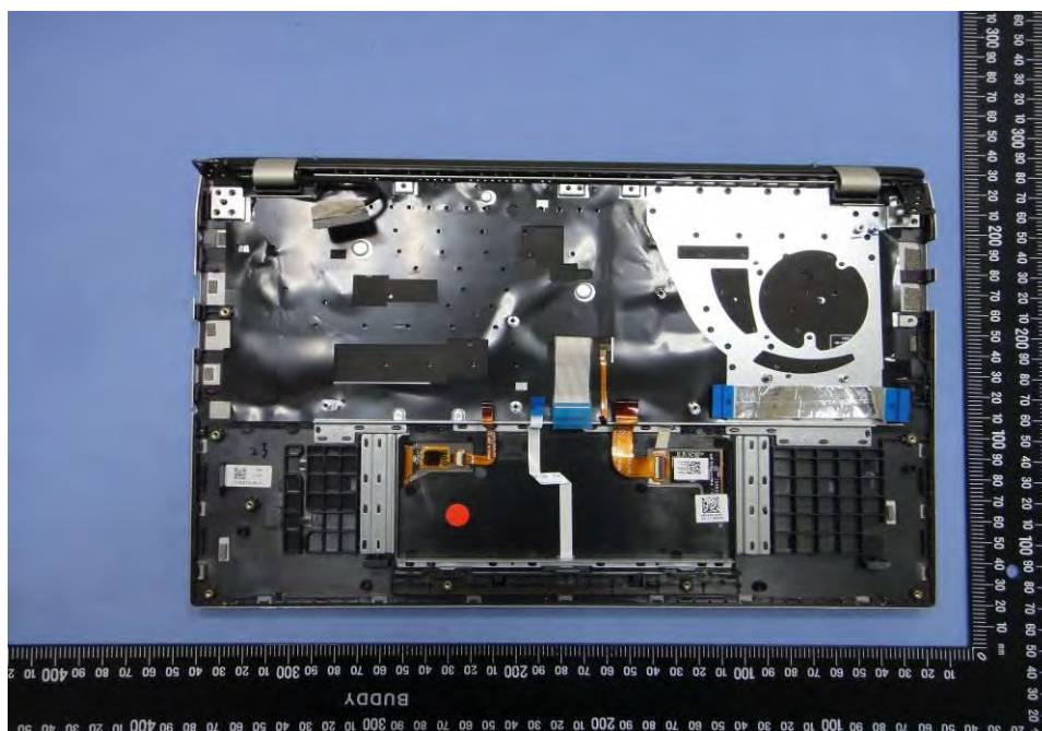
EUT Photo (66)
