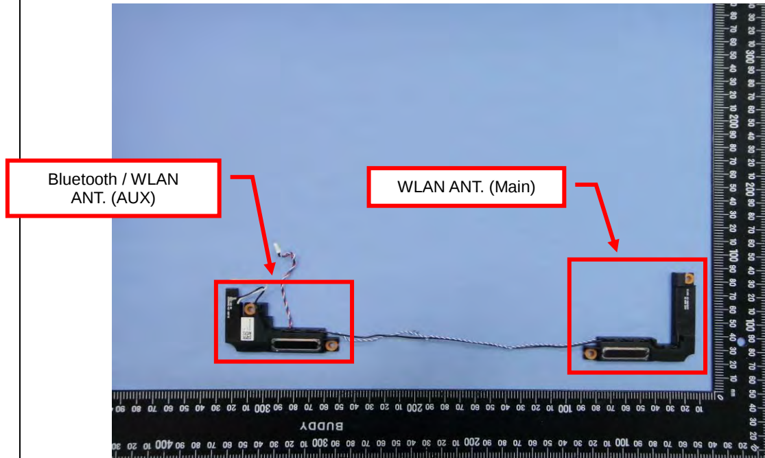
EUT Photo (62)
