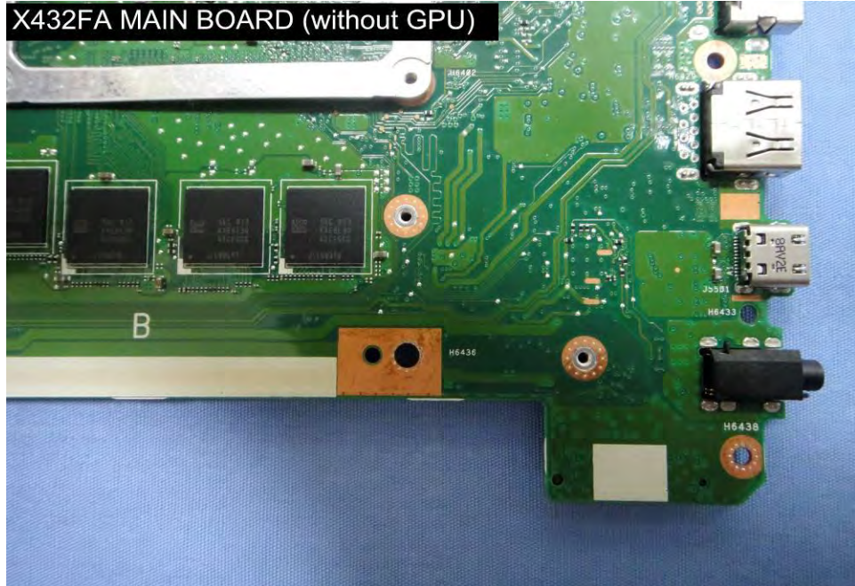
EUT Photo (50)
