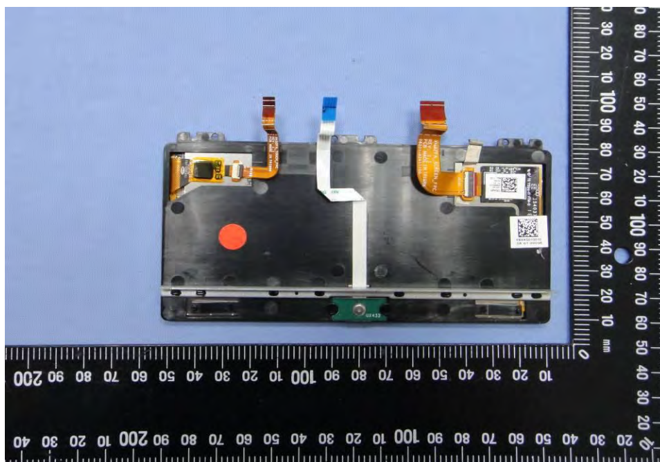
EUT Photo (66)
