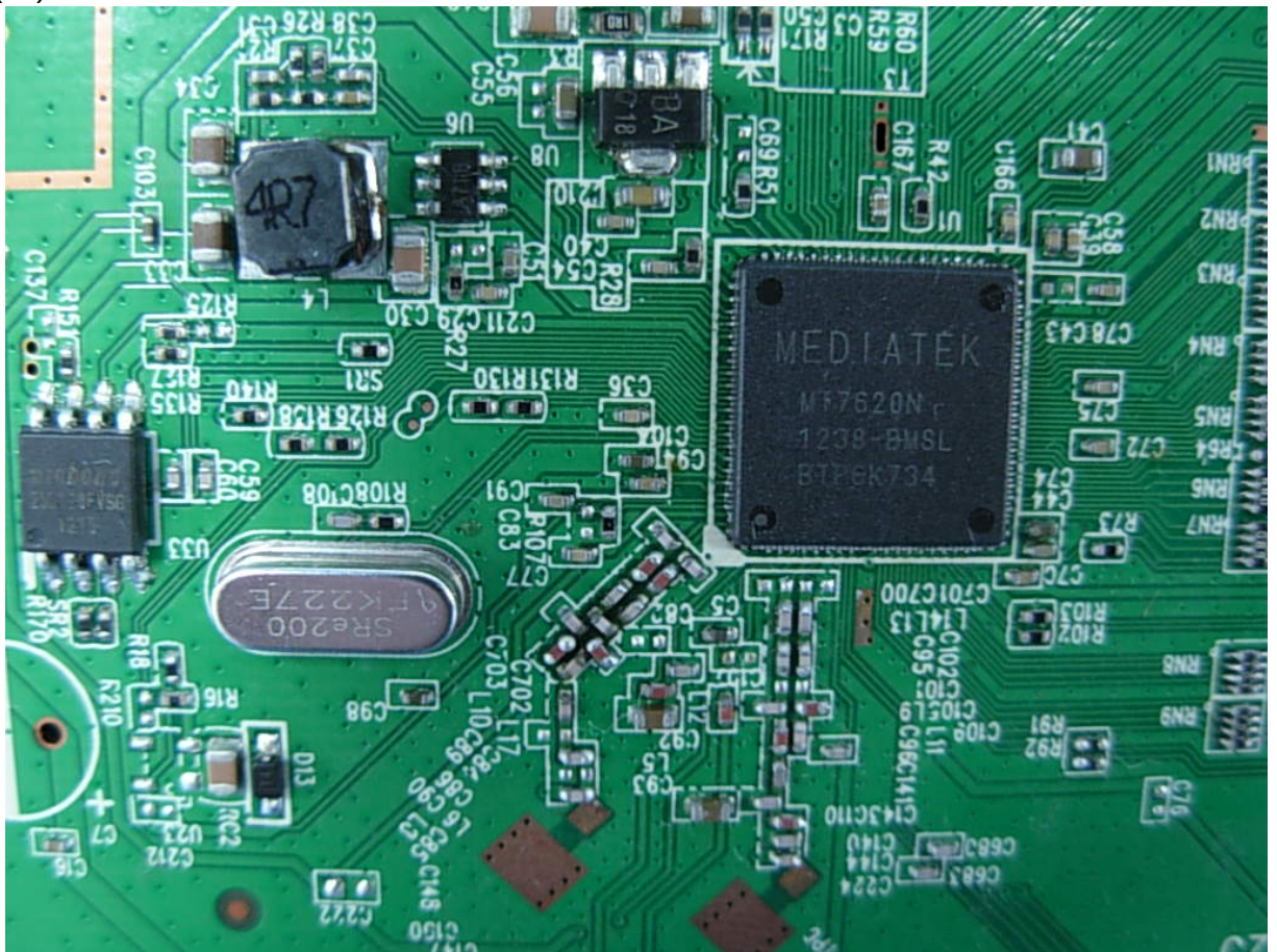
(12) EUT Photo
