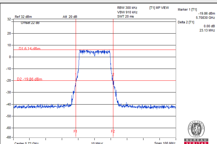
802.11be (EHT20) Beamforming / Chain 2 : CH 144 (U-NII-3)
