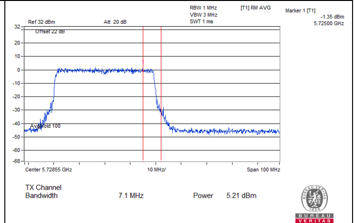
802.11be (EHT40) Beamforming / Chain 3 : CH 142 (U-NII-3)
