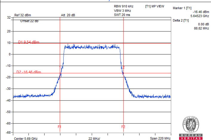
802.11be (EHT80) Beamforming / Chain 0 : CH 138 (U-NII-3)
