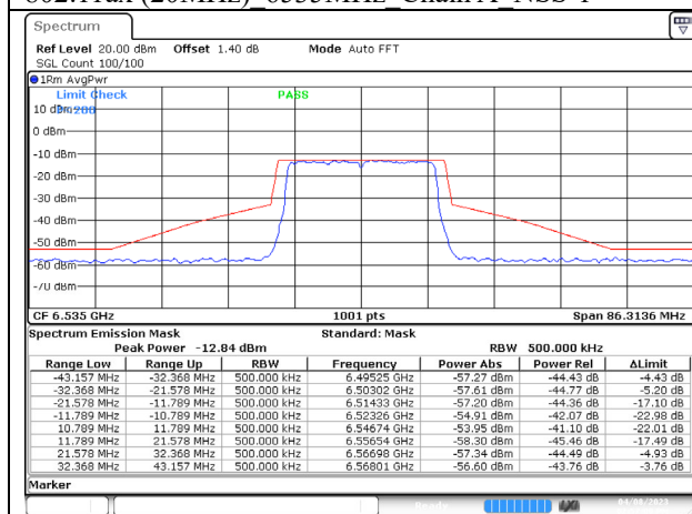
802.11ax (20MHz) 6535MHz Chain A NSS-1
