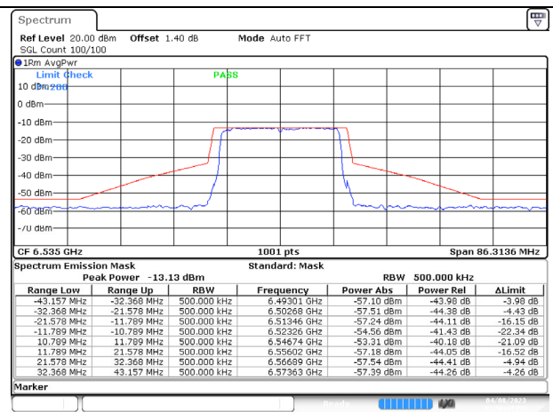
802.11ax (20MHz) 6535MHz Chain B NSS-1
