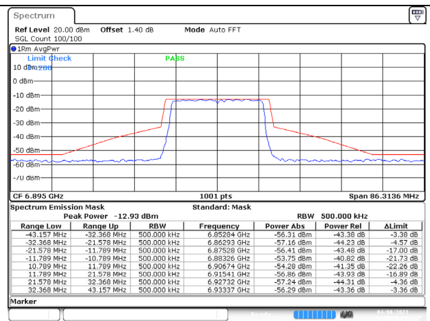
802.11ax (20MHz) 6895MHz Chain D NSS-1
