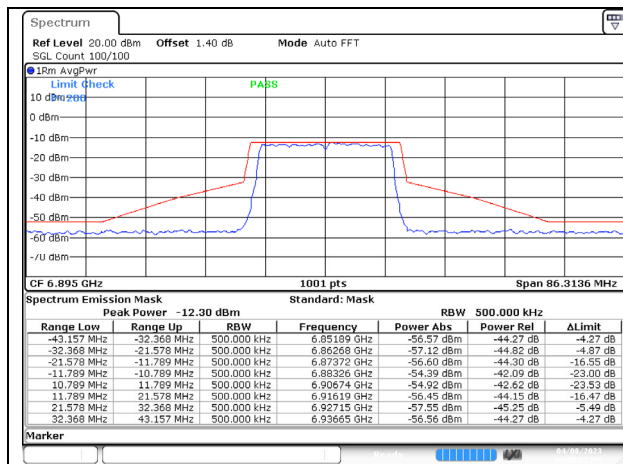
802.11ax (20MHz) 6895MHz Chain C NSS-1
