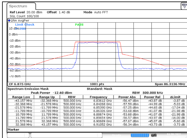
802.11ax (20MHz) 6875MHz Chain A NSS-1
