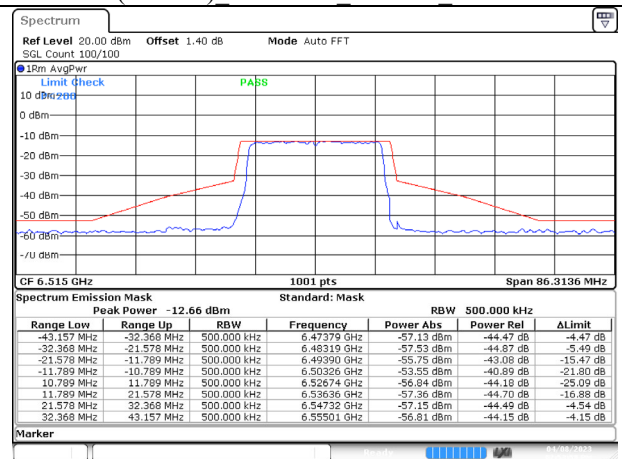
802.11ax (20MHz) 6515MHz Chain B NSS-1
