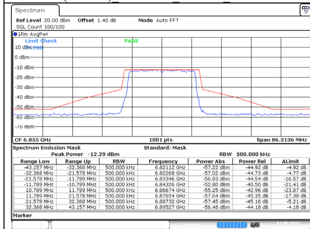
802.11ax (20MHz) 6855MHz Chain A NSS-1
