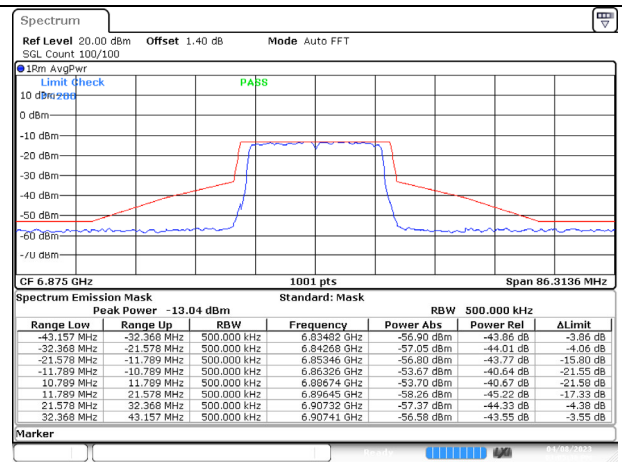
802.11ax (20MHz) 6875MHz Chain B NSS-1
