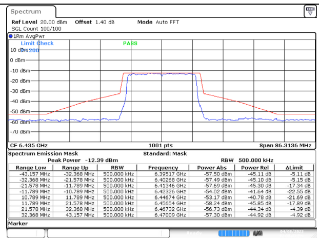
802.11ax (20MHz) 6435MHz Chain B NSS-1
