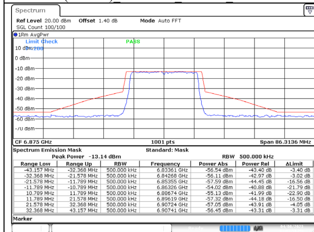
802.11ax (20MHz) 6875MHz Chain A NSS-1
