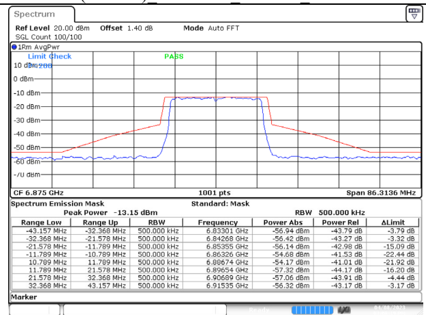
802.11ax (20MHz) 6875MHz Chain B NSS-1
