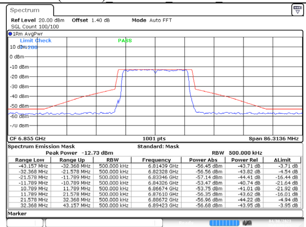
802.11ax (20MHz) 6855MHz Chain B NSS-1
