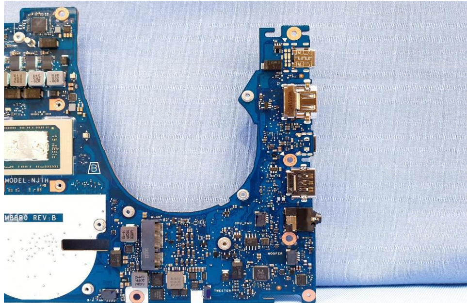
EUT Photo (13)
