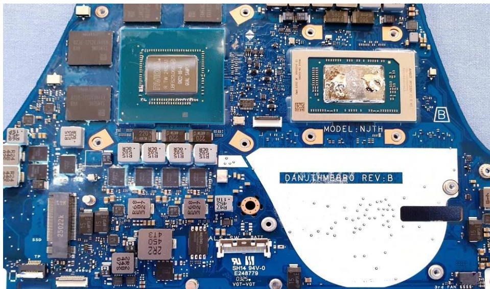
EUT Photo (12)
