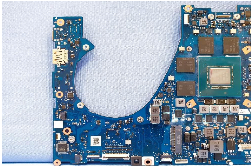
EUT Photo (12)
