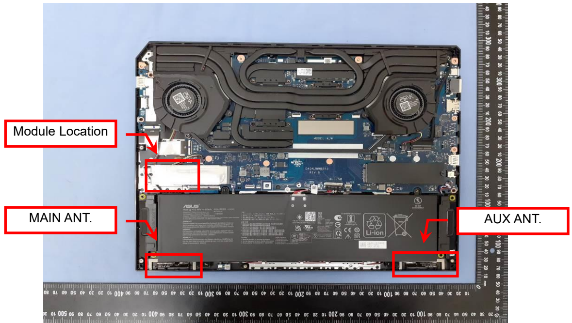
EUT Photo (2)
