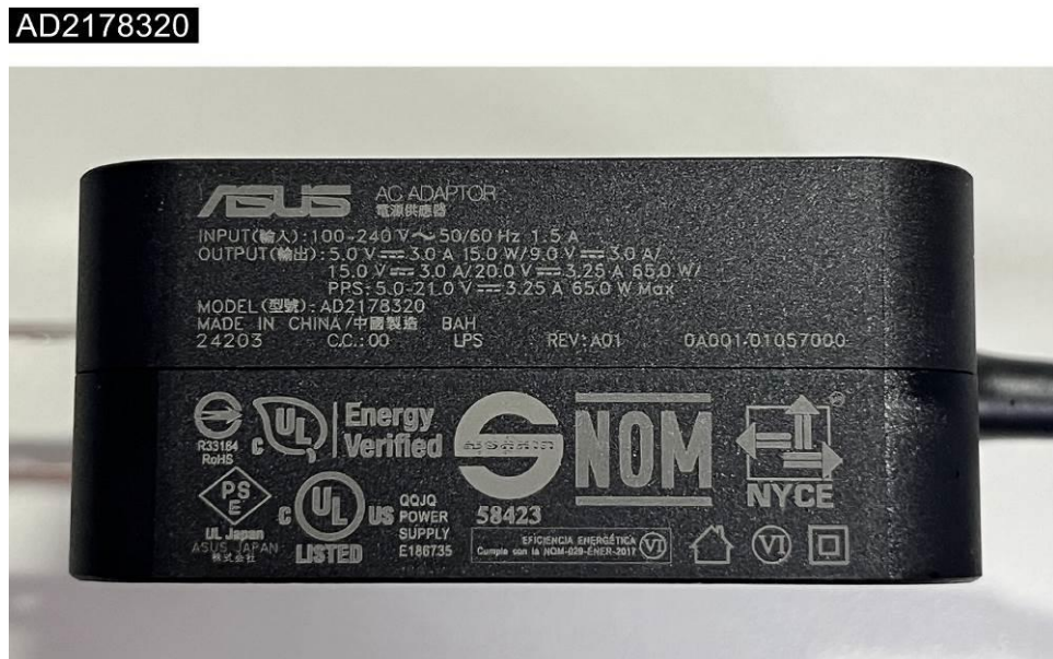
EUT Photo (14)
