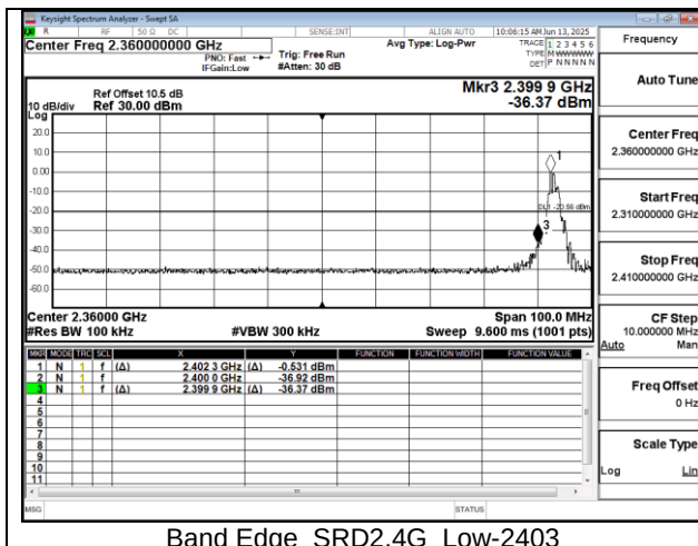
Band Edge SRD2.4G Low-2403
