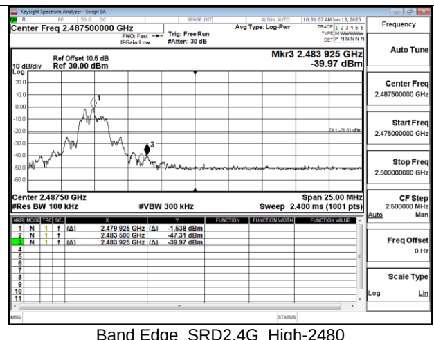
Band Edge SRD2.4G High-2480
