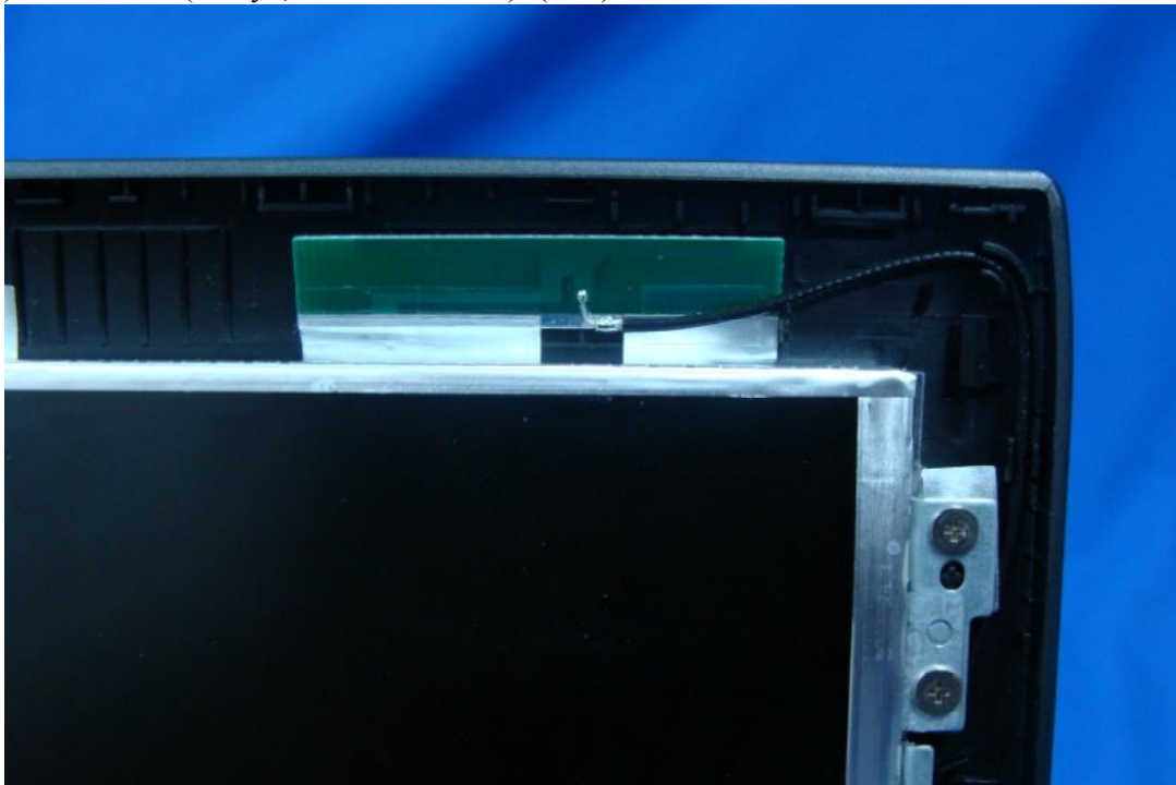
(16) EUT Photo (Whyu, C660-520271-A)- (Aux)
