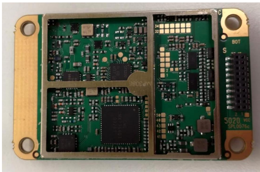
Bottom
