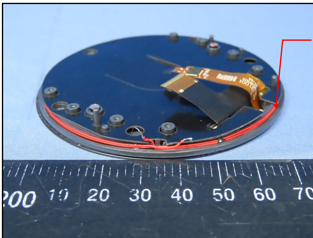
NFC Antenna
