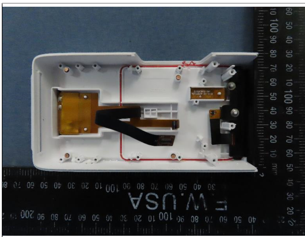
ANT2 (NFC)
