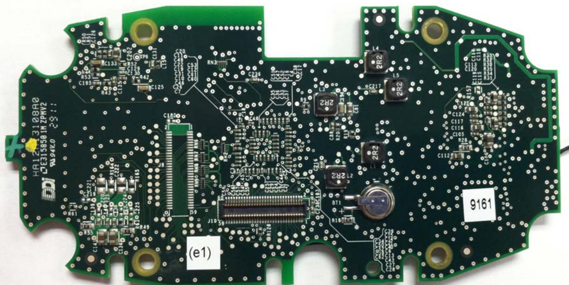
TAP801-01 PCB - Bottom
