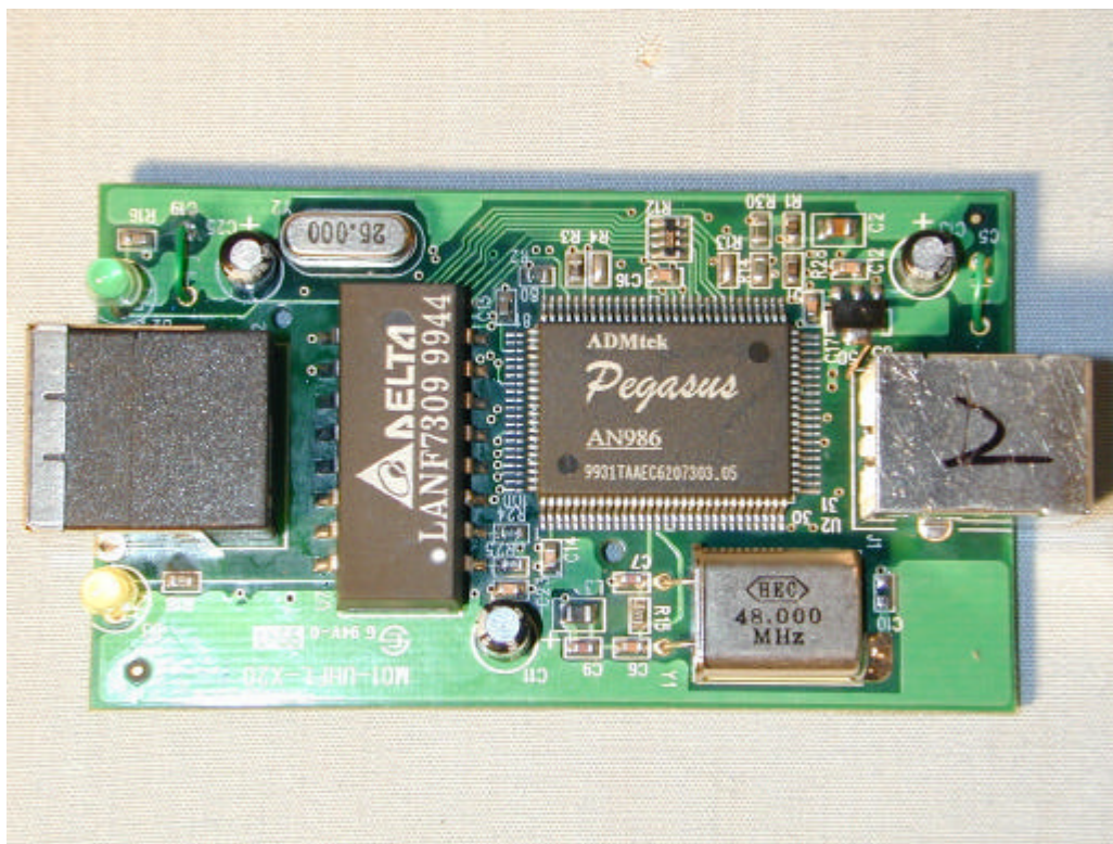
(4) EUT Photo
