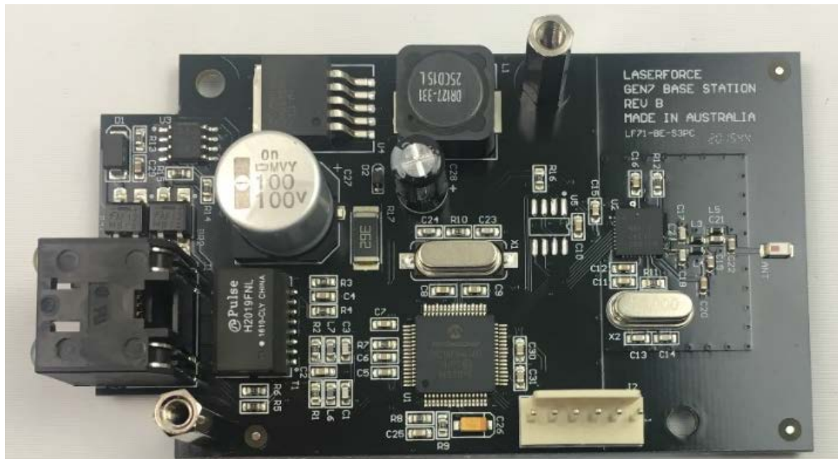
PCB Top
